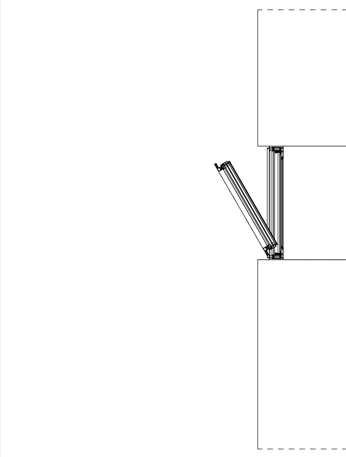
VE10 1 220cmx60cm 1 folha oscilo-batente Abertura para exterior Caixilharia em aluminio lacado cinza com folha em vidro duplo incolor
