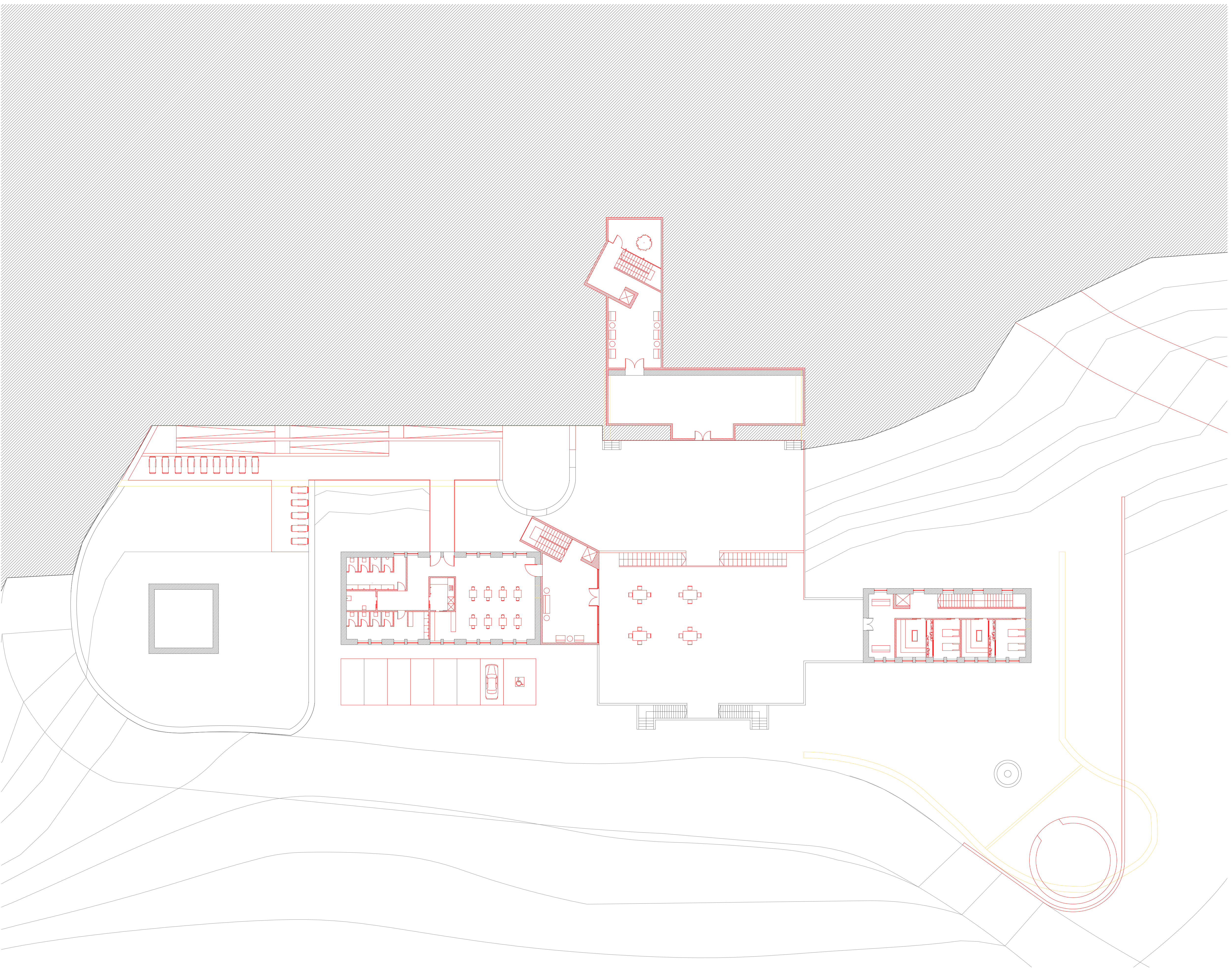
"Re-habitar as Termas Radium" Cláudia Vanessa Marques Gonçalves Planta de Vermelhos e Amarelos Desenho 15 Escala 1/200 Orientadora - Prof. Doutora Inês Daniel de Campos Co-orientadora - Prof. Doutora Cláudia Sofia Beato Universidade da Beira Interior novembro 2019
