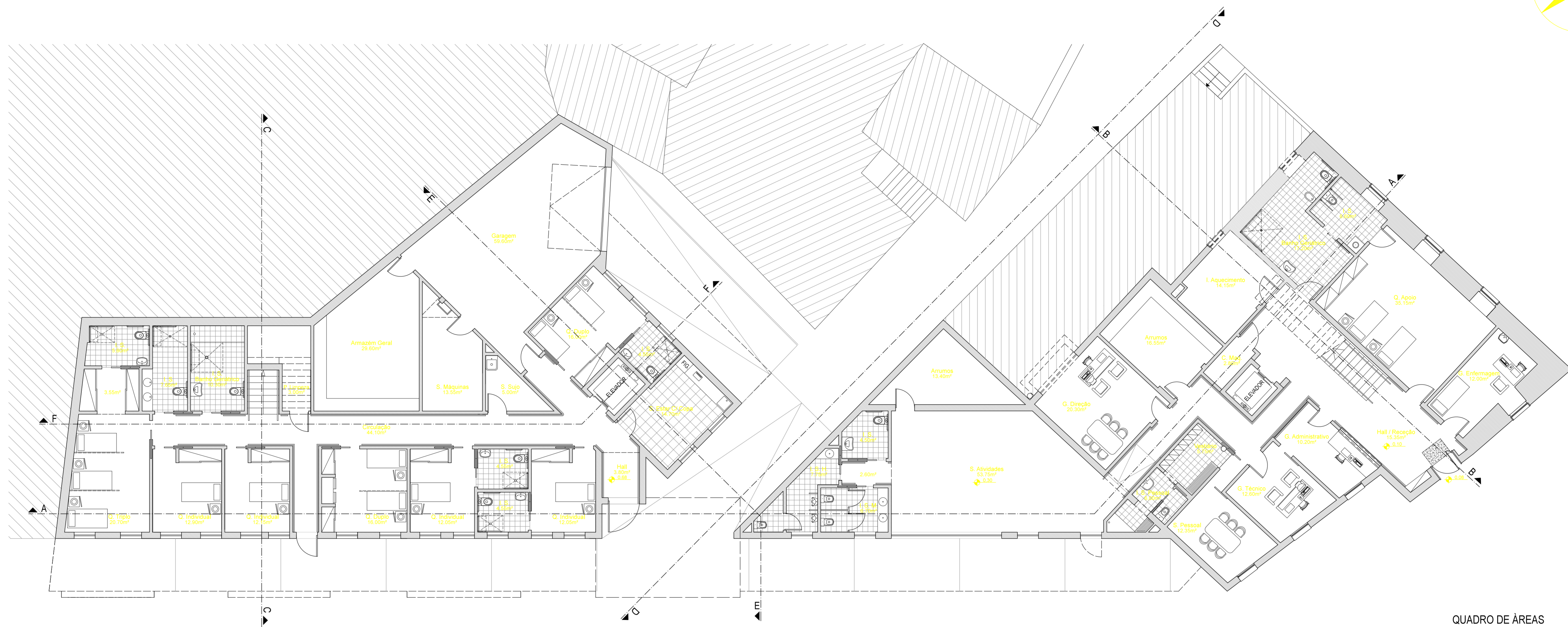
PLANTA DO PISO 0 PROPOSTO
