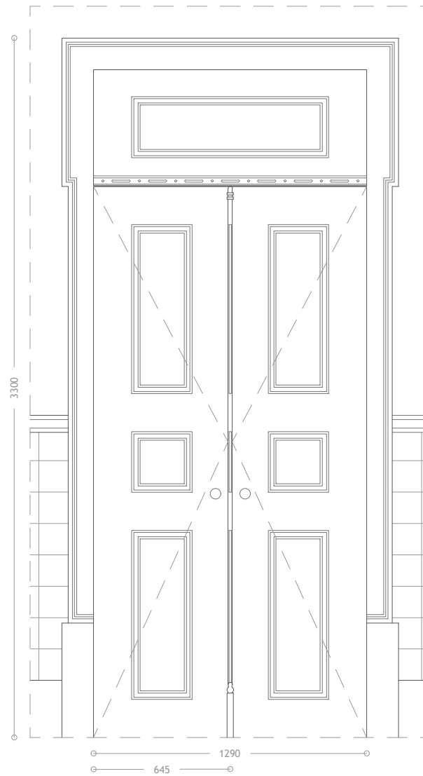
Imagem 183 - Levantamento gráfico da Porta P4 - Frente - Escala 1:25
