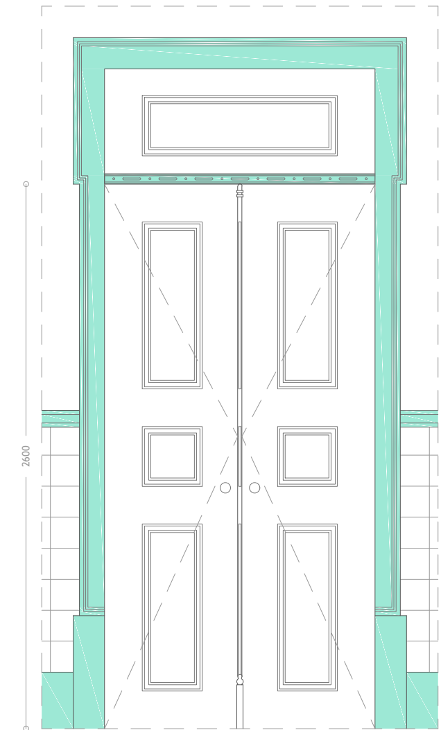
Imagem 184 - Levantamento gráfico a cores da Porta P4 - Frente - Escala 1:25
