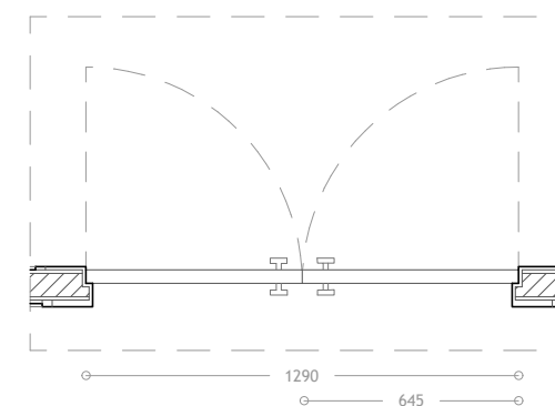
Imagem 185 - Levantamento gráfico da Porta P4 - Planta - Escala 1:25
