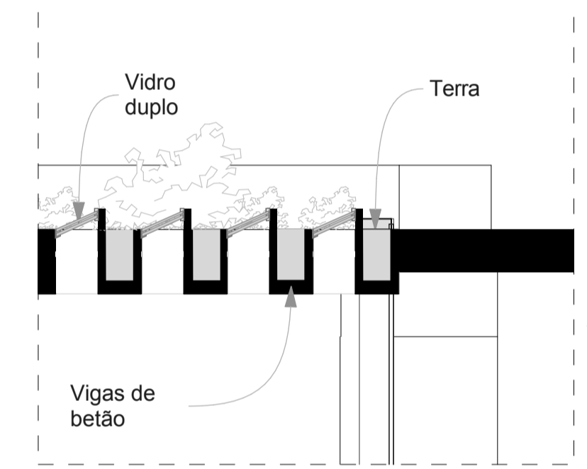
Detalhe D-01 1:25
