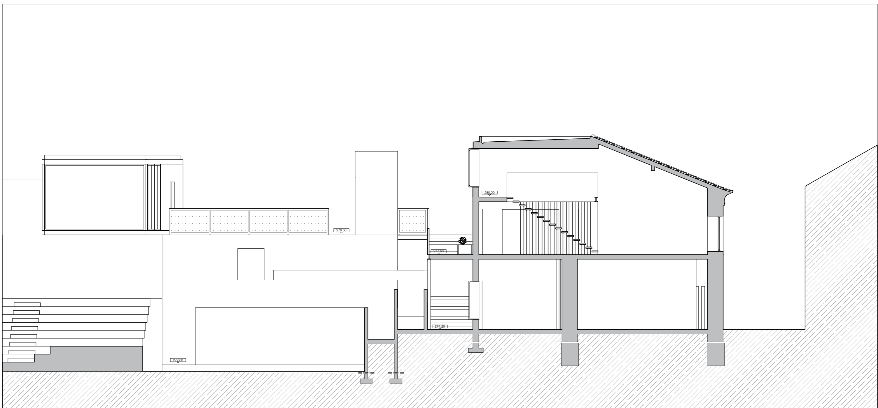
CORTE S2 ANEXOS CASA PINA FALCÃO
