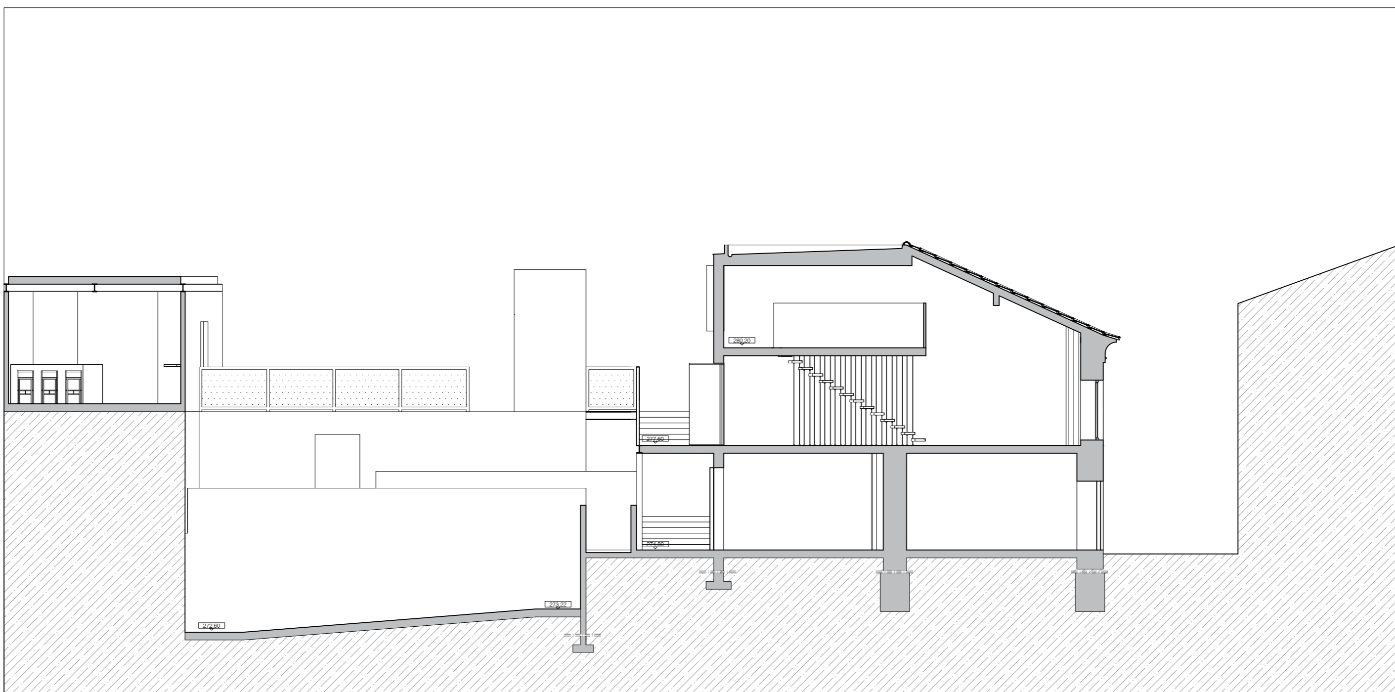
CORTE S3 ANEXOS CASA PINA FALCÃO
