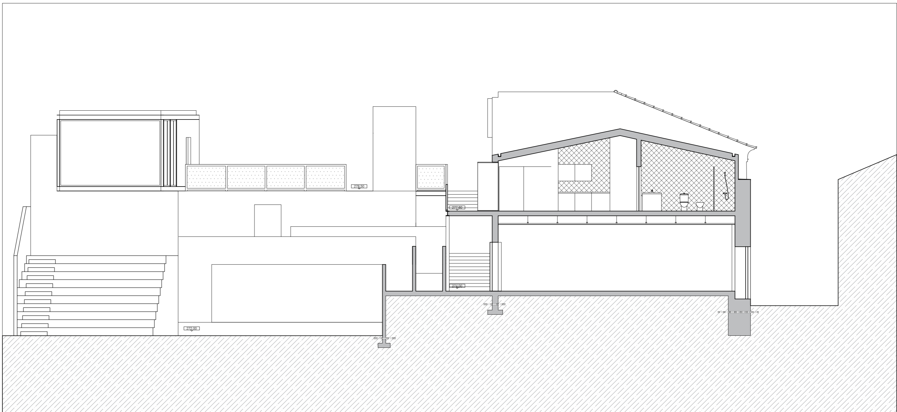
CORTE S1 ANEXOS CASA PINA FALCÃO
