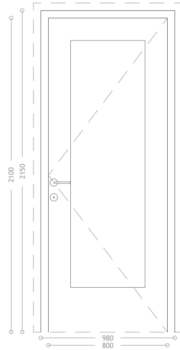
Imagem 282 - Levantamento gráfico da Porta P14 - Frente - Escala 1:25
