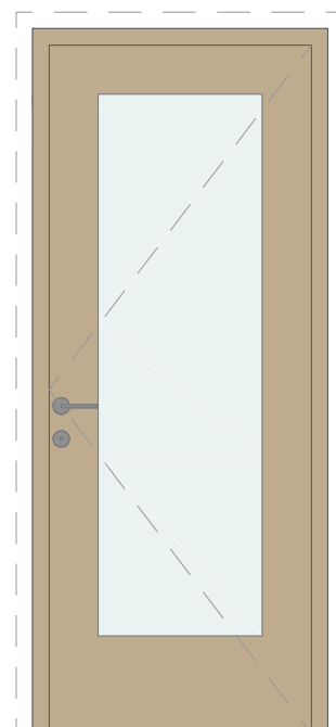
Imagem 284 - Levantamento gráfico a cores da Porta P14 - Frente - Escala 1:25
