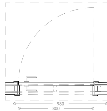
Imagem 283 - Levantamento gráfico da Porta P14 - Planta - Escala 1:25
