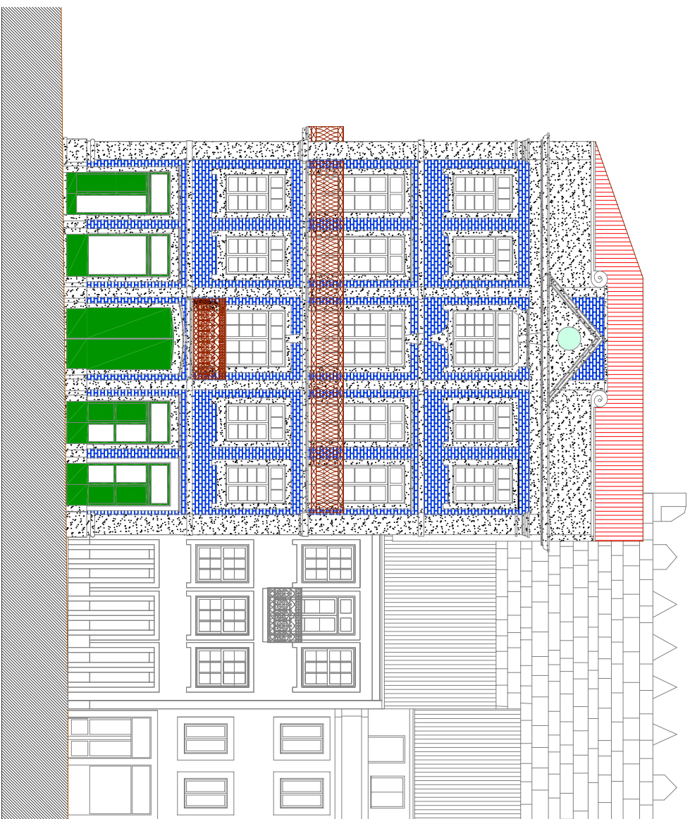
ALÇADO PRINCIPAL
