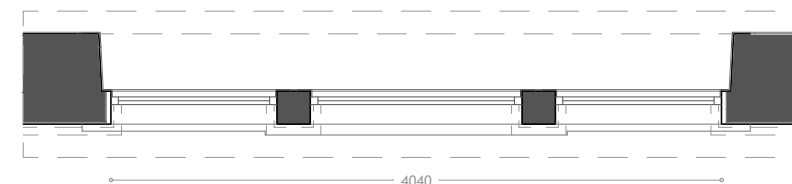
Imagem 222 - Levantamento gráfico da Janela V6 - Planta - Escala 1:50
