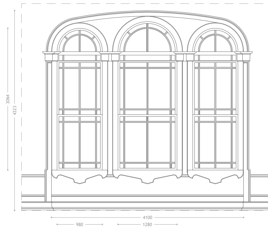
Imagem 221 - Levantamento gráfico da Janela V6 - Interior - Escala 1:50
