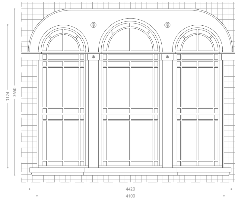
Imagem 220 - Levantamento gráfico da Janela V6 - Exterior - Escala 1:50
