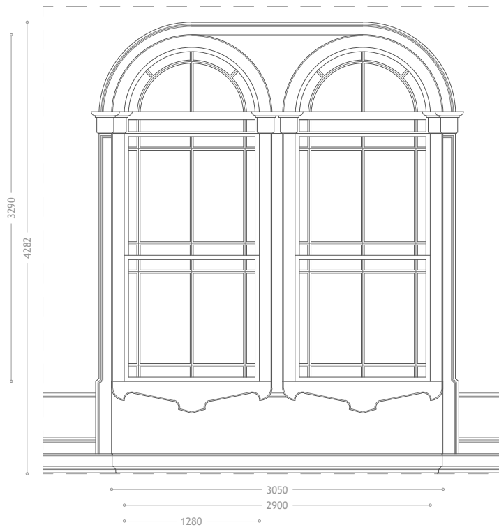
Imagem 230 - Levantamento gráfico da Janela V7 - Interior - Escala 1:50
