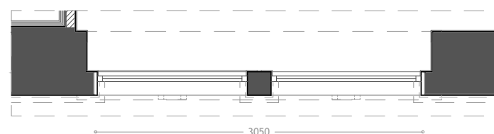
Imagem 231 - Levantamento gráfico da Janela V7 - Planta - Escala 1:50
