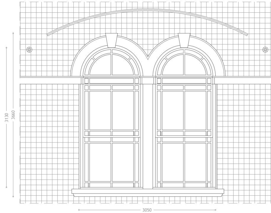
Imagem 229 - Levantamento gráfico da Janela V7 - Exterior - Escala 1:50
