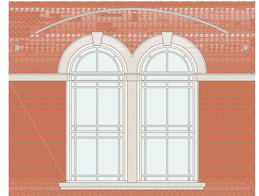
Imagem 232 - Levantamento gráfico a cores da Janela V7 - Exterior - Escala 1:50
