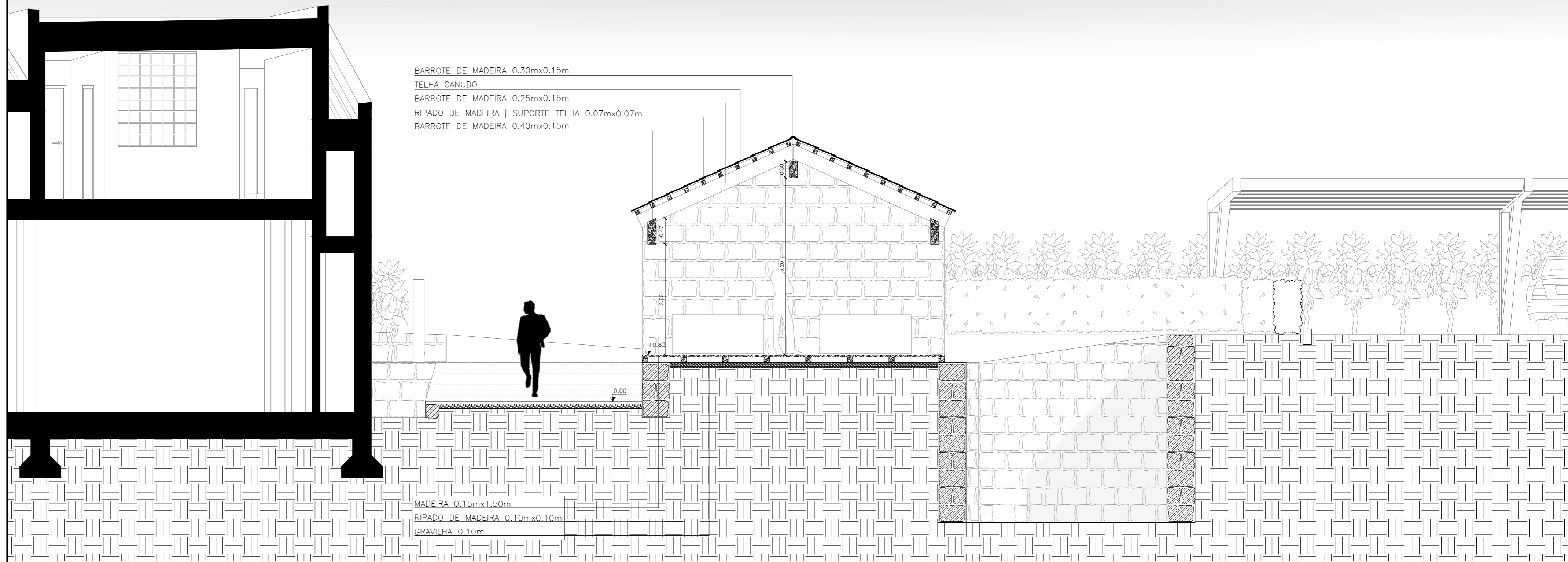
CORTE C|C' ESCALA 1:50
