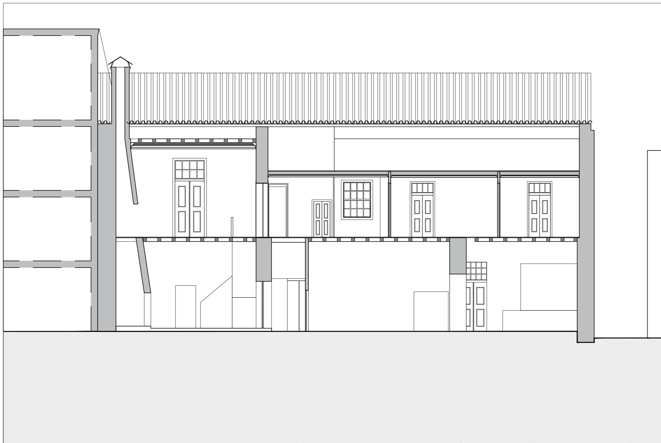
CORTE S1 CASA PINA FALCÃO
