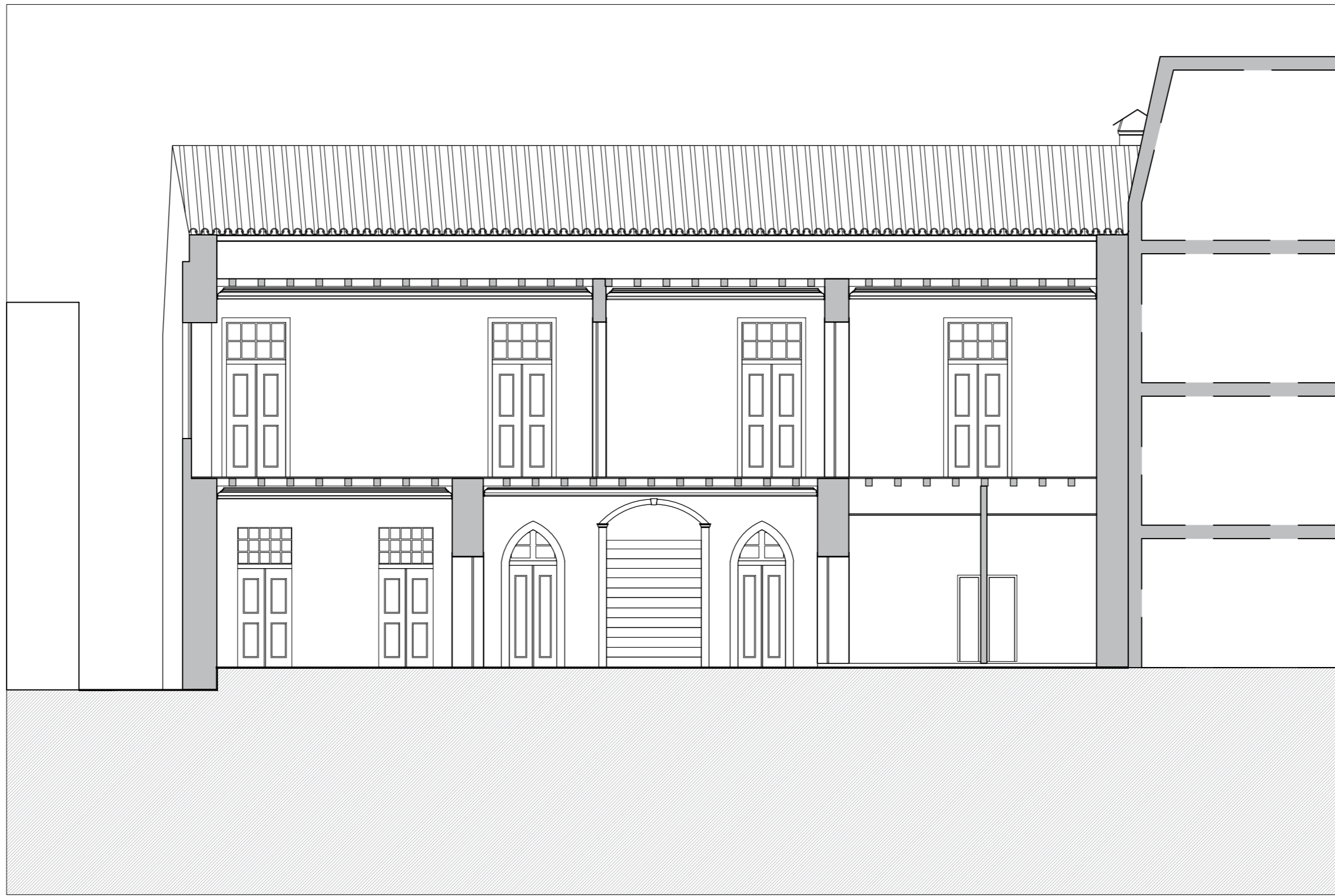
CORTE N1 CASA PINA FALCÃO
