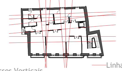
Esquema de Acessos Verticais
