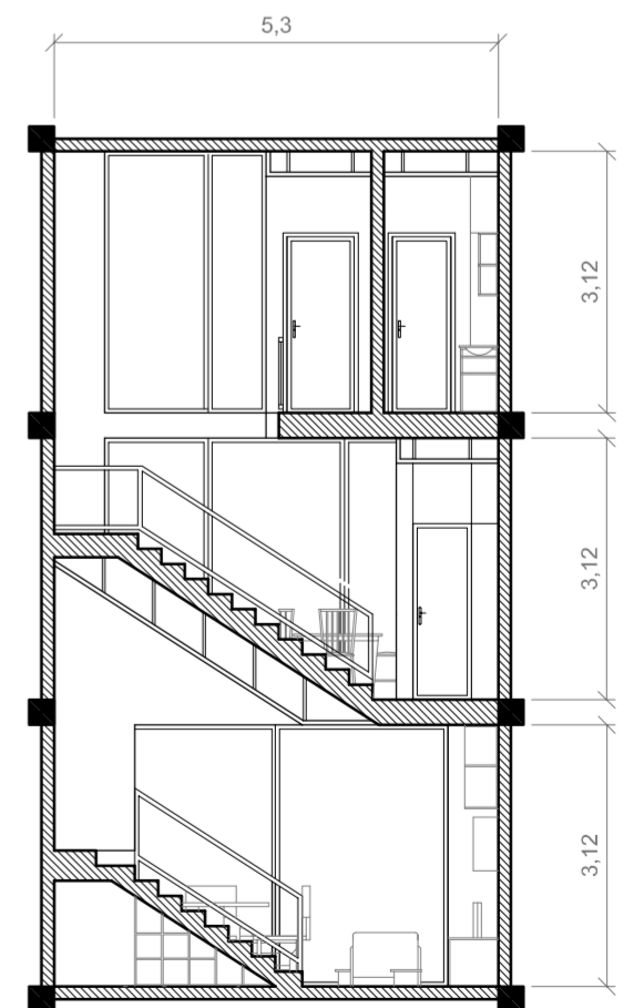
Corte DD'
