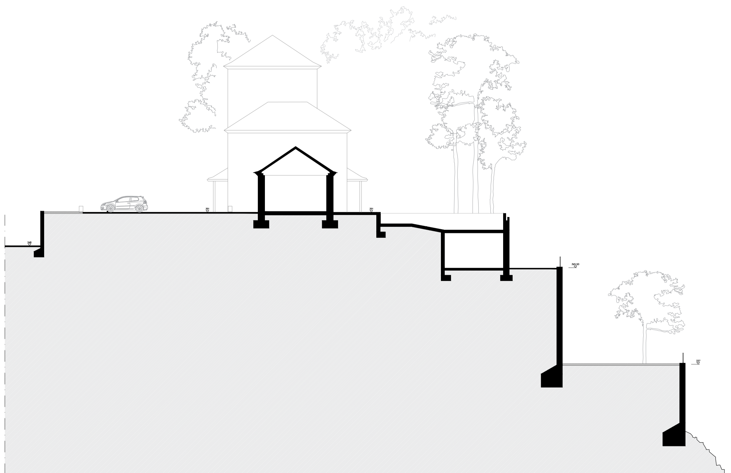
Corte CC
