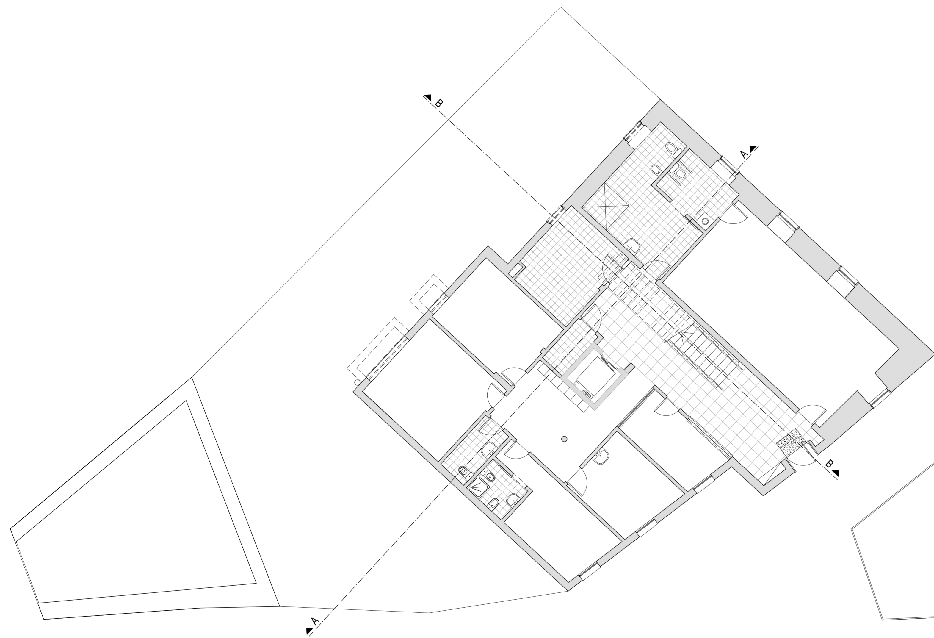
PLANTA DO PISO 0 EXISTENTE
