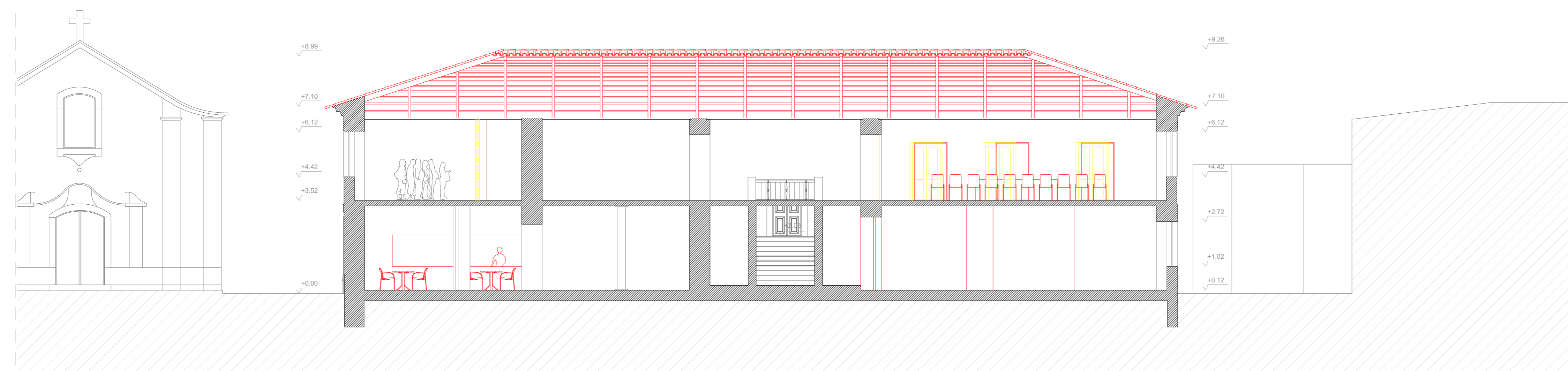
CORTE TRANSVERSAL C
