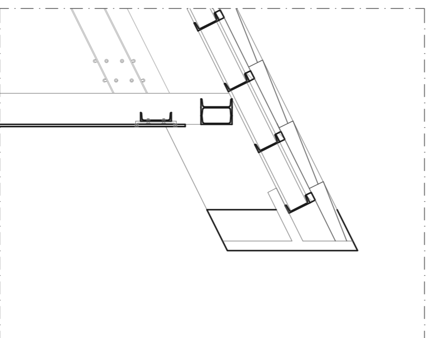
Planta da Cobertura 1/20
