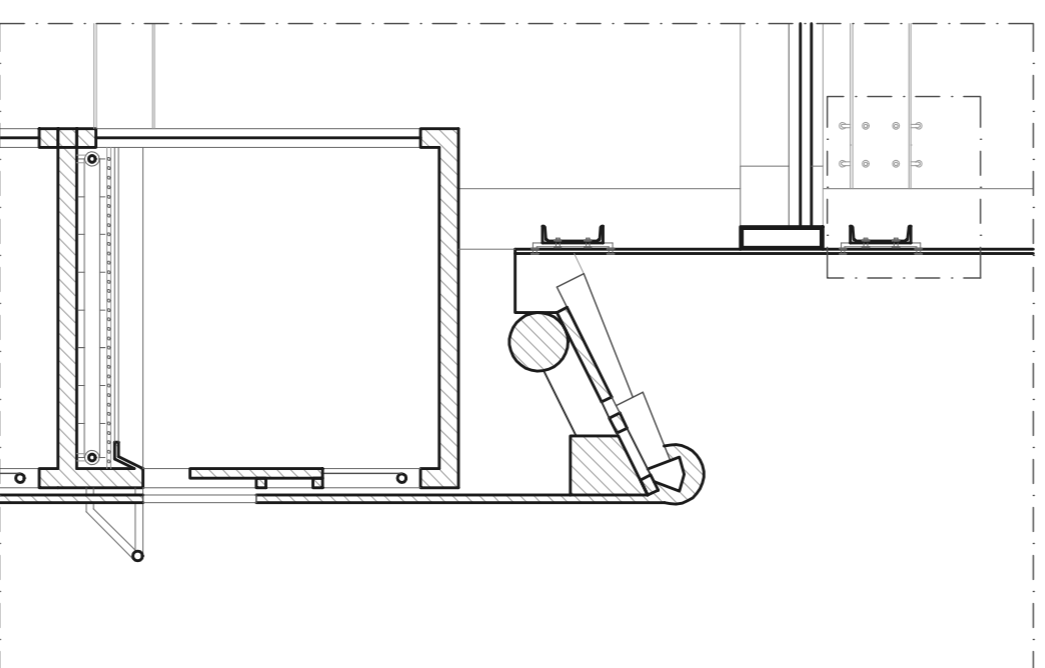
Planta da Cobertura 1/20
