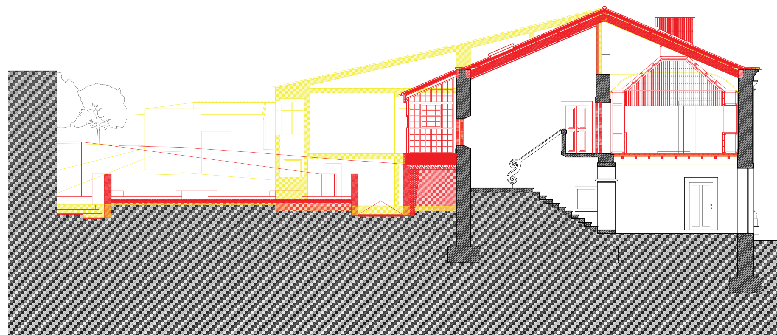
CORTE AA'
