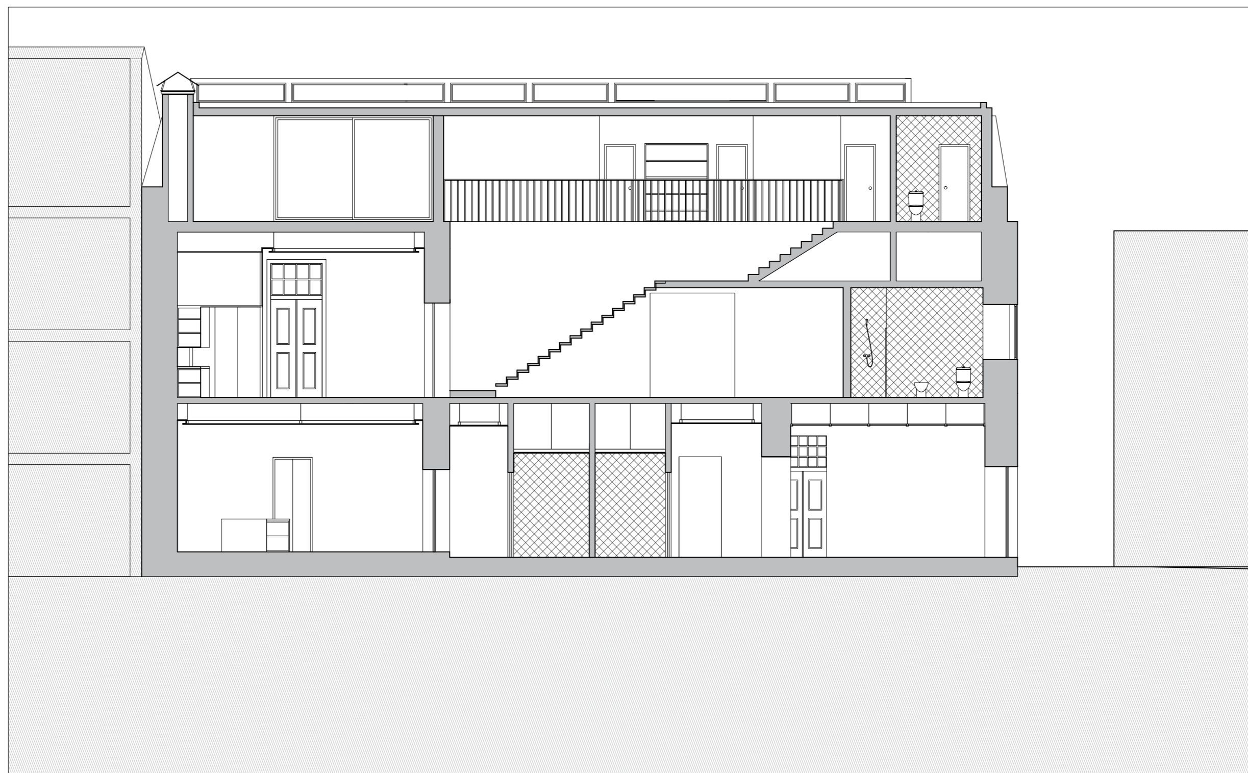
CORTE S1 CASA PINA FALCÃO
