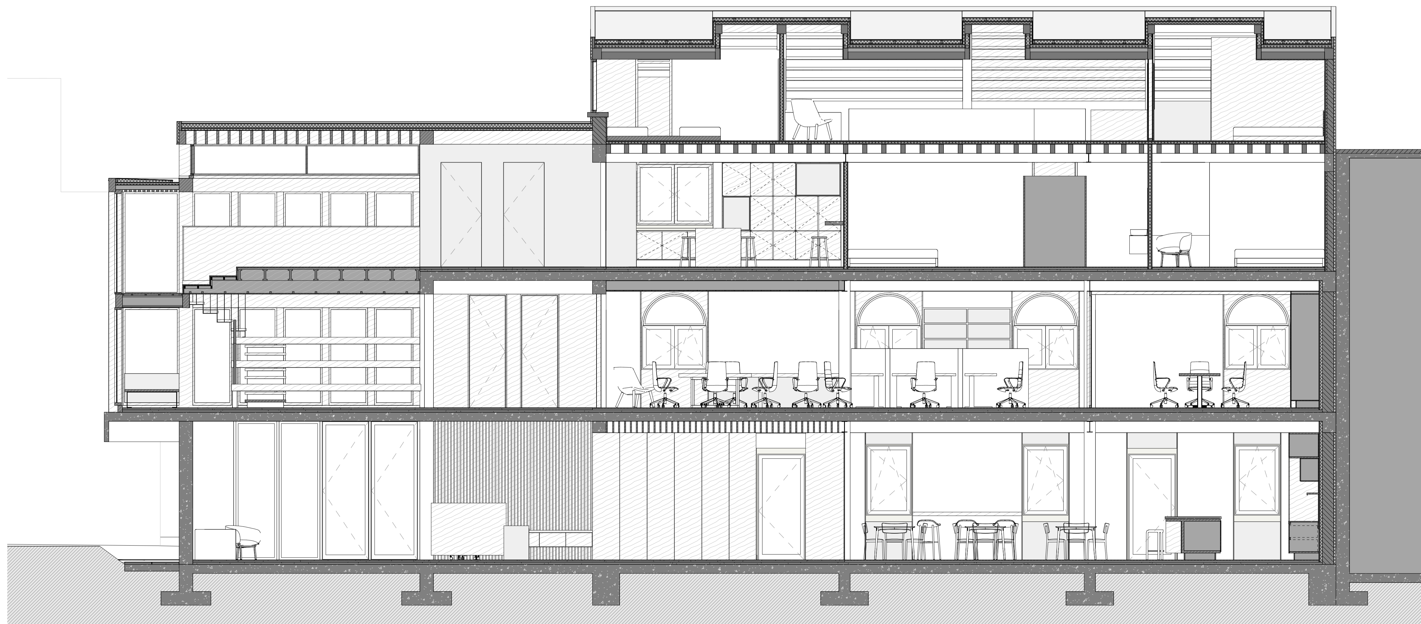
CORTE B
