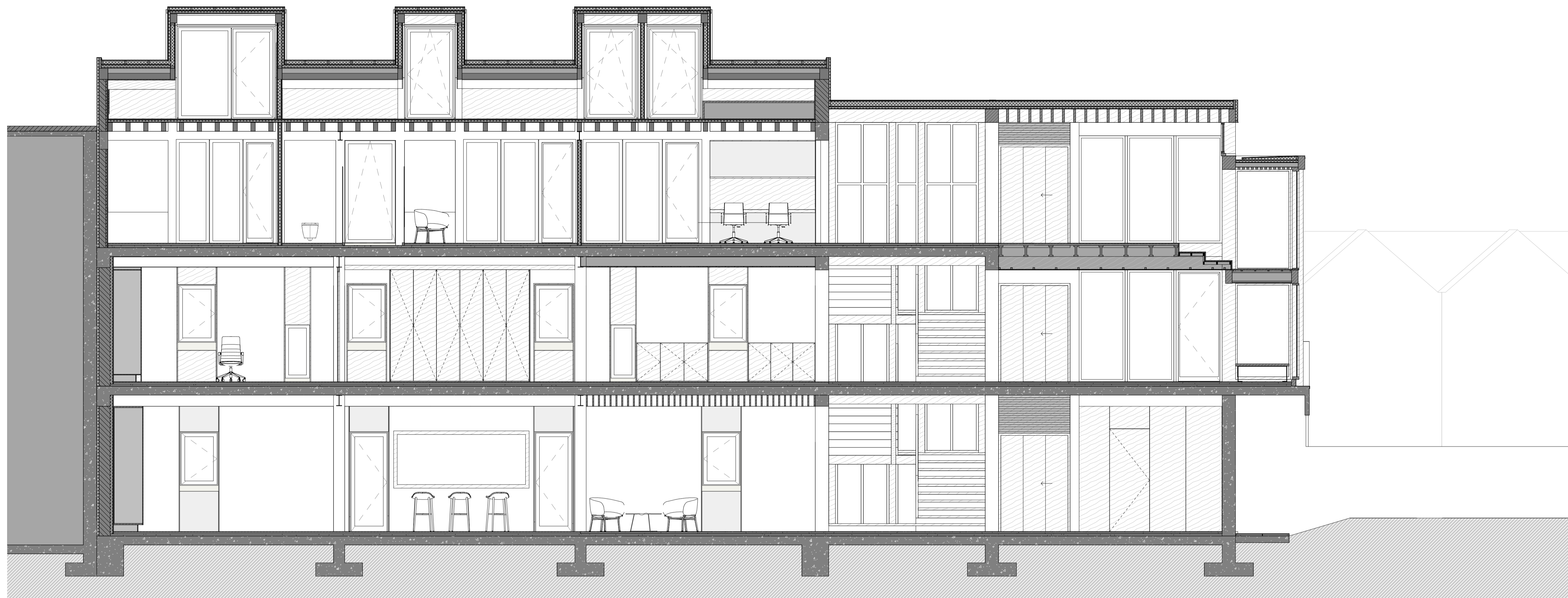
CORTE A
