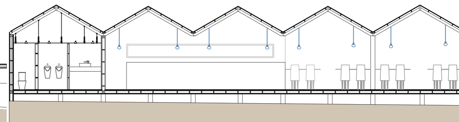
Corte CC'
