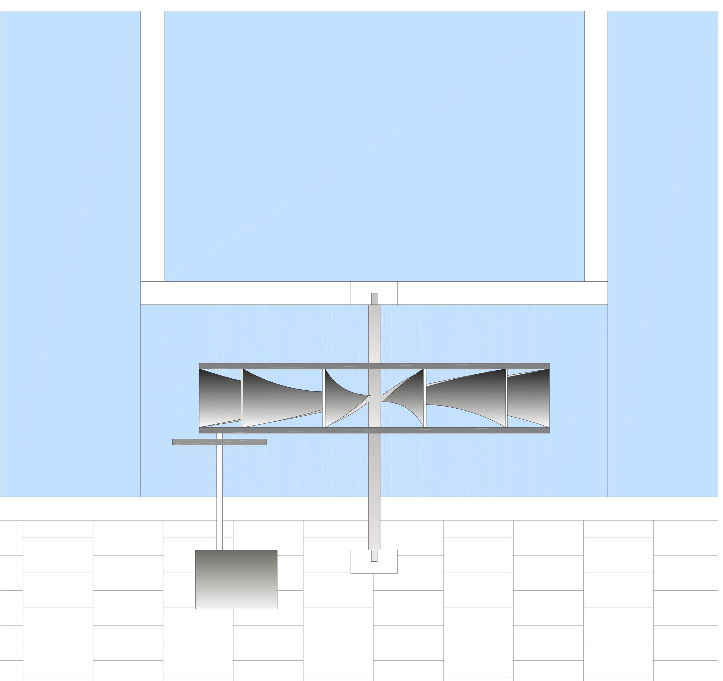
Planta
