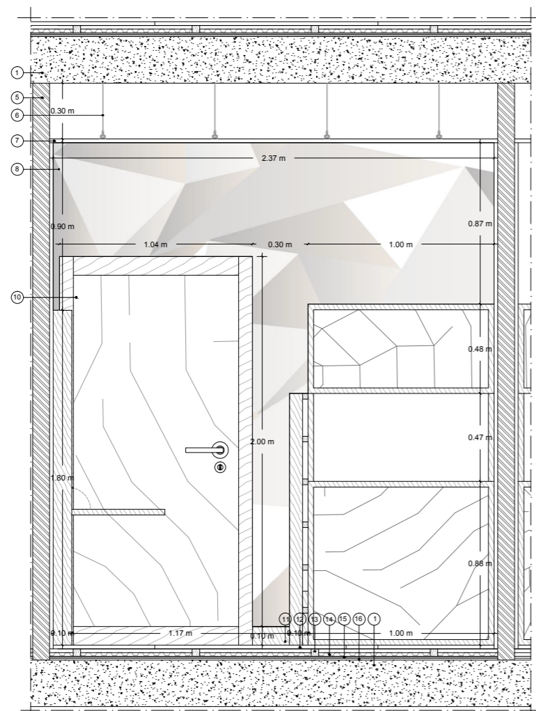
Corte CC'
