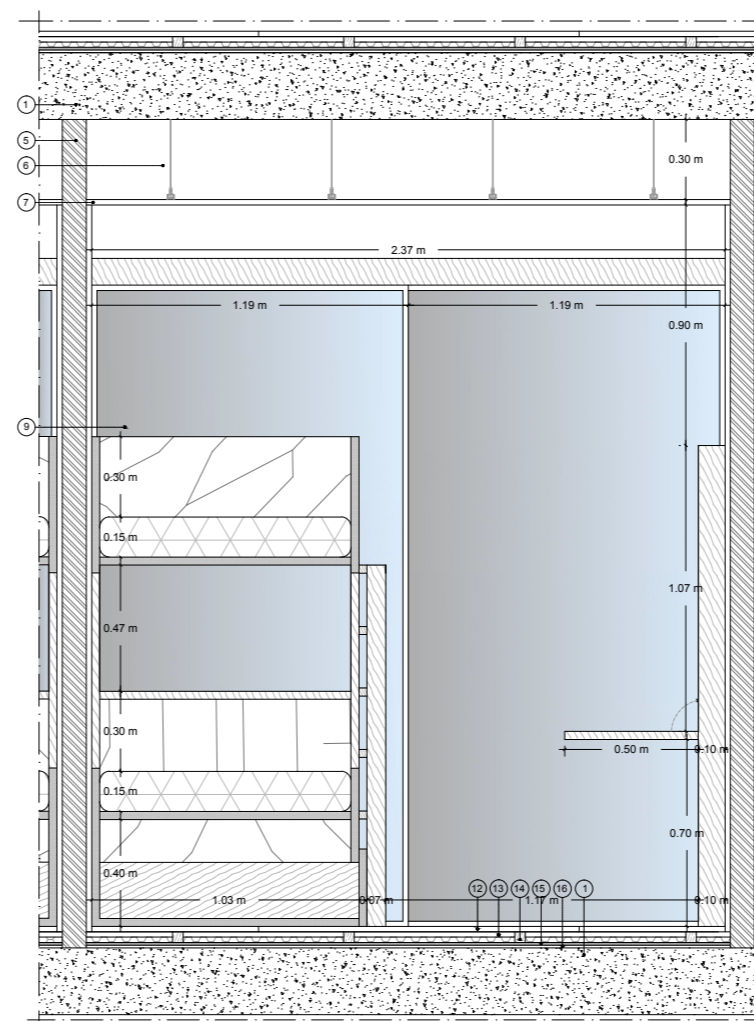
Corte DD'
