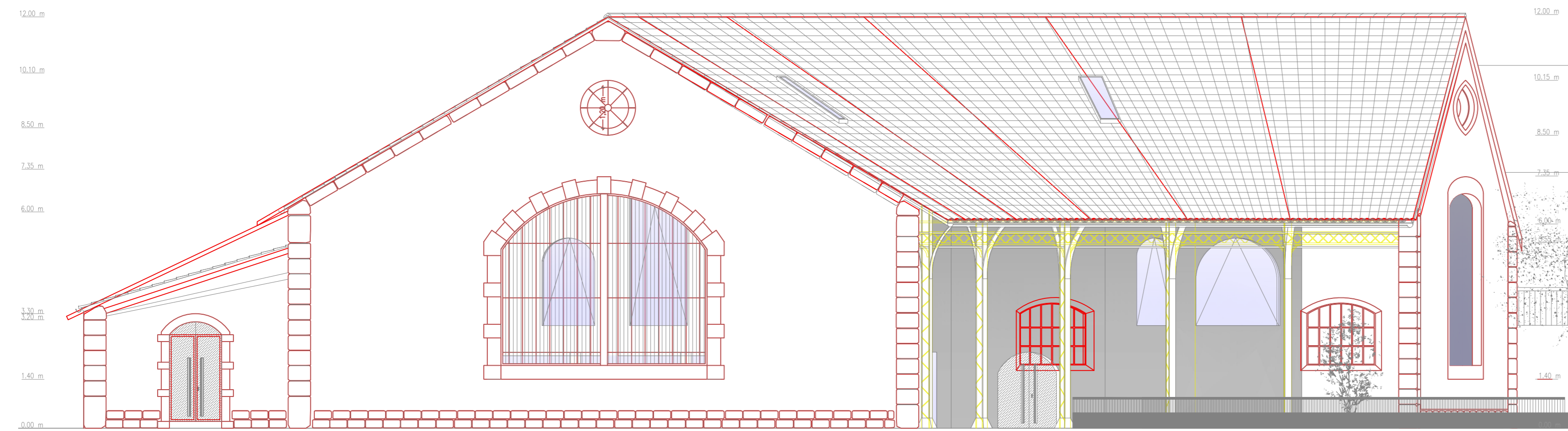
ALÇADO NORTE
