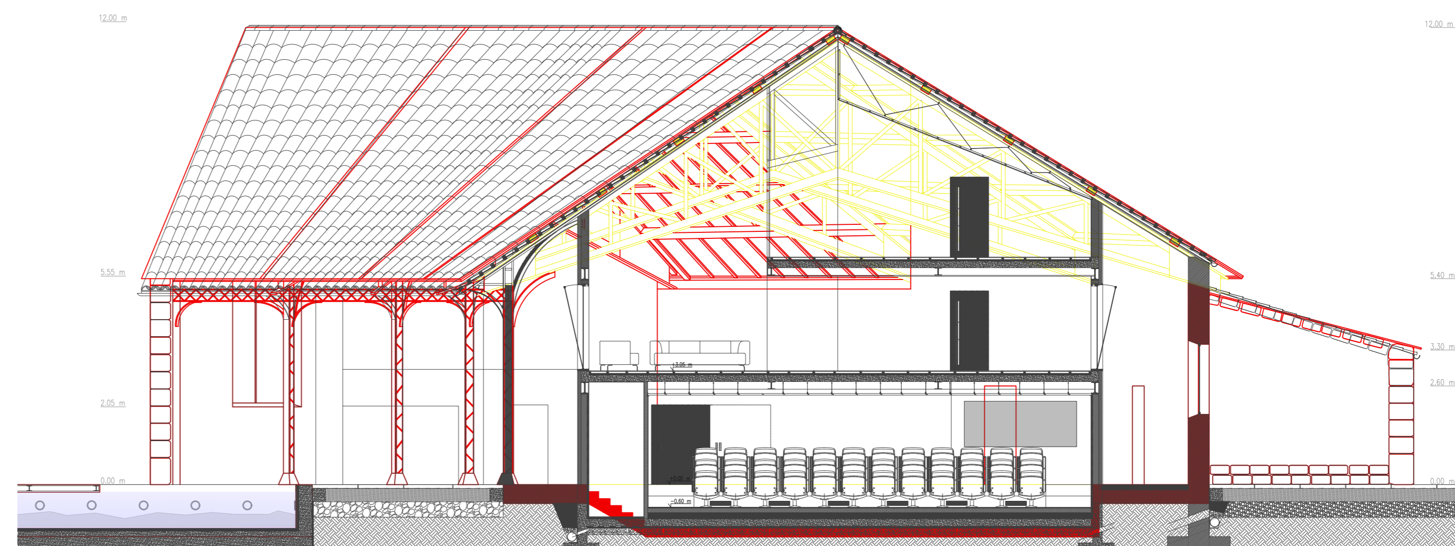
CORTE AA'
