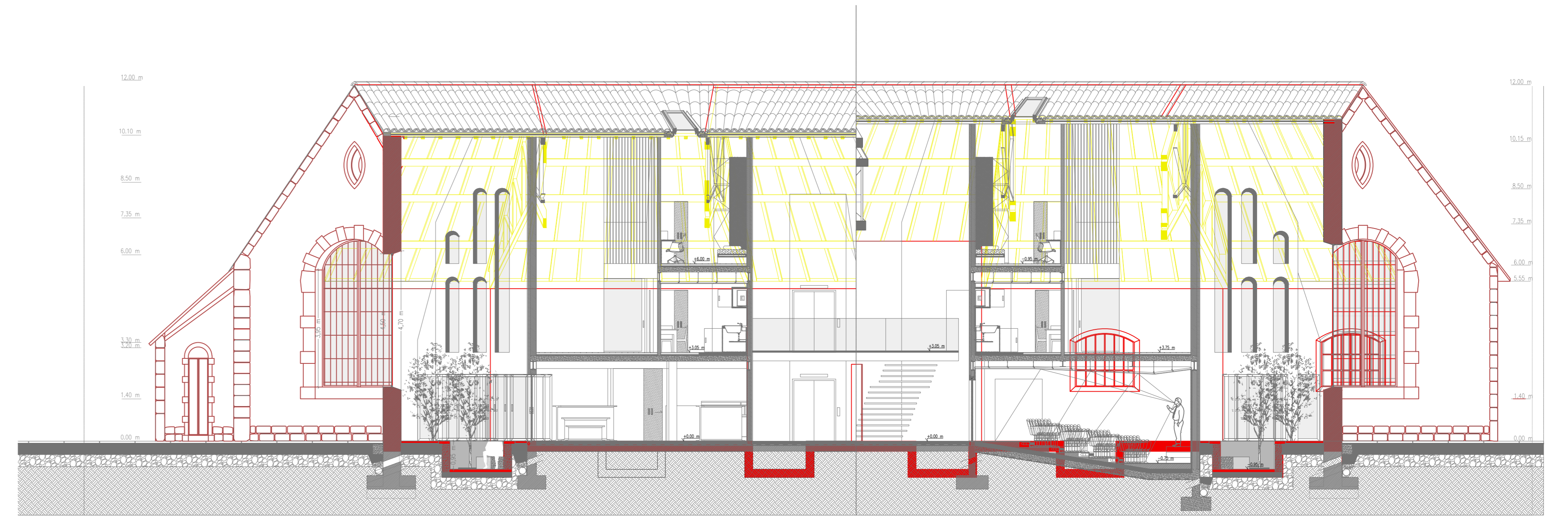
CORTE CC'
