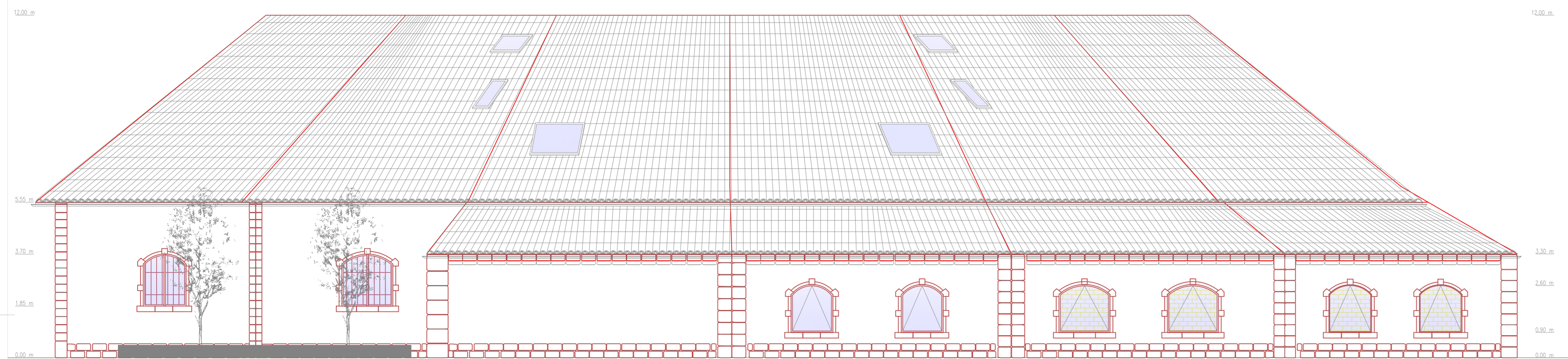
ALÇADO ESTE
