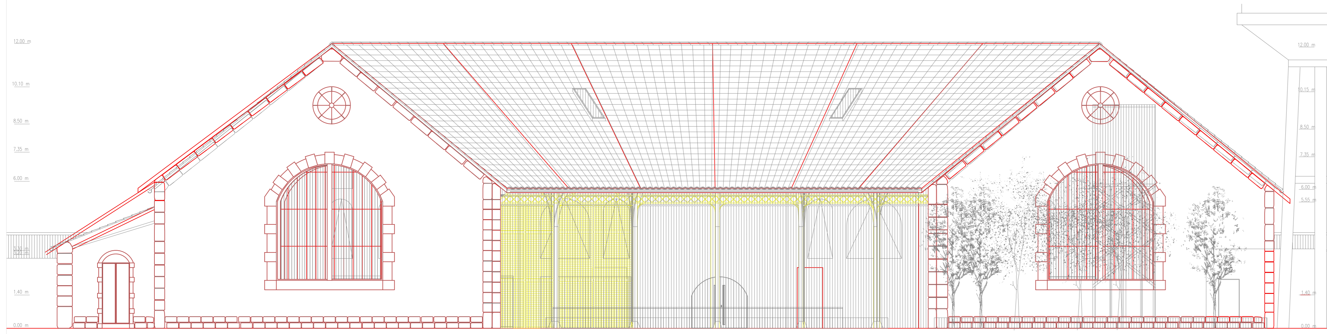
ALÇADO OESTE
