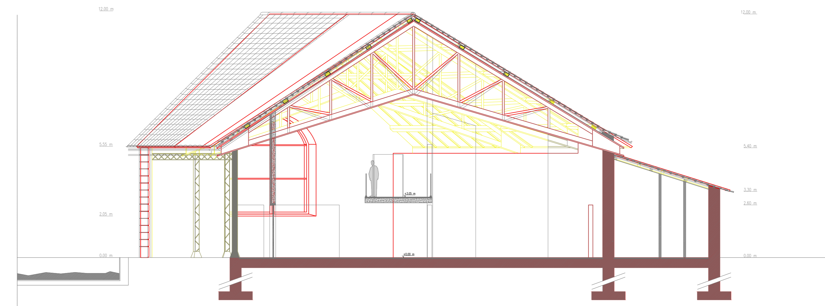
CORTE DD'
