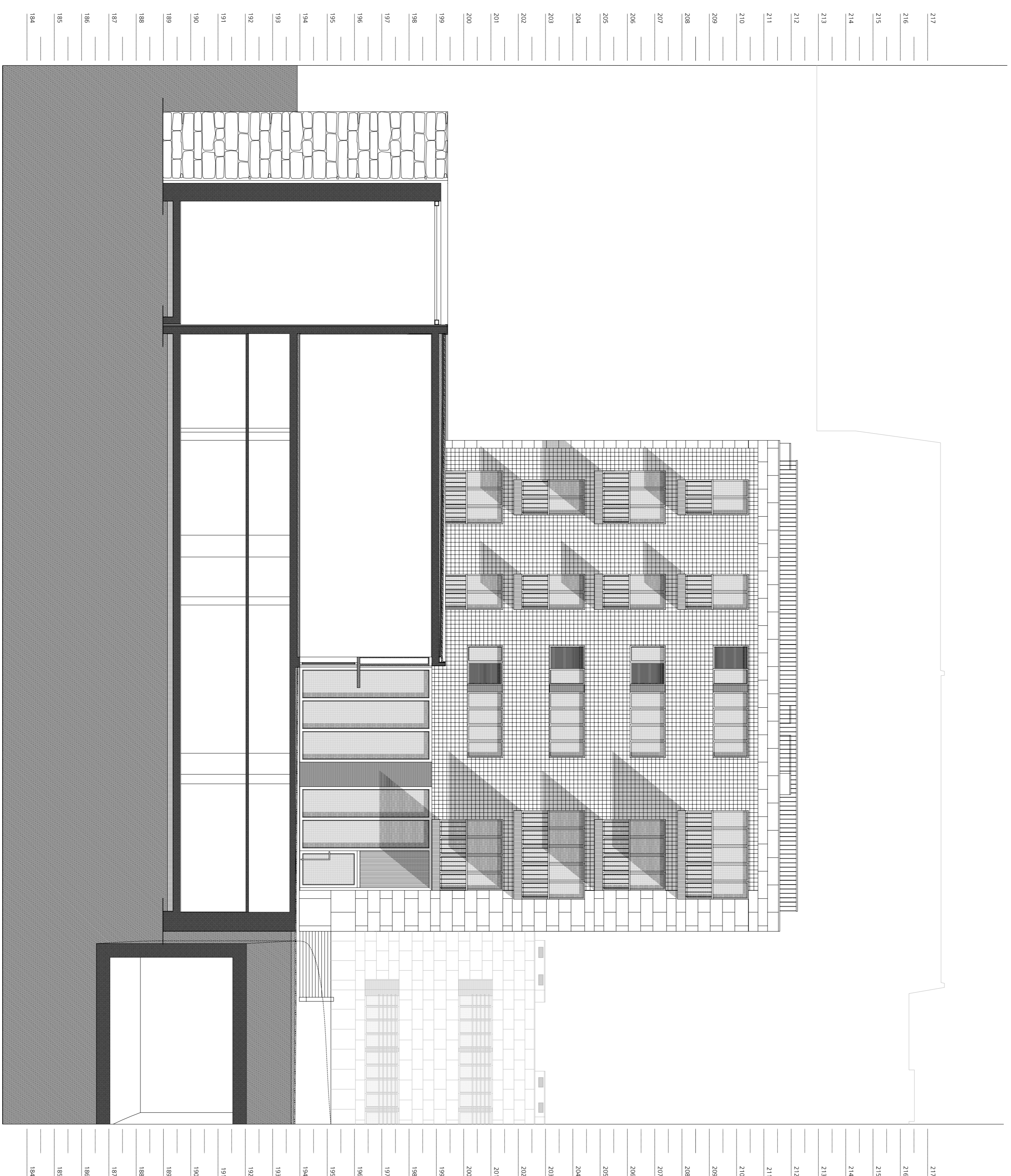
EDIFICIO C - alçado Poente / corte DD
