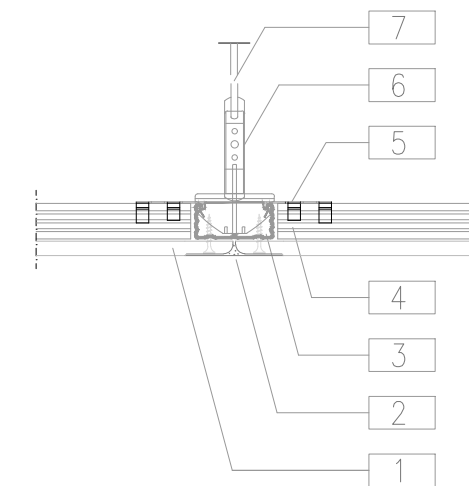
Pormenor de juntas longitudinal, sobre borde BA
