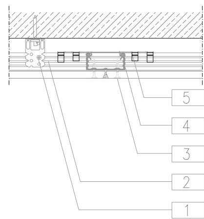
Pormenor de ancoragem directa, junta transversal
