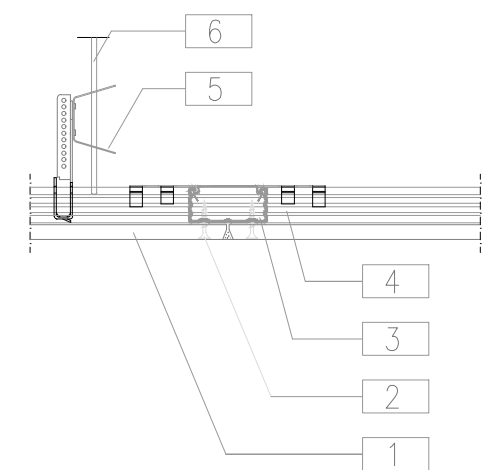
Pormenor de juntas transversal, cantos Biselados
