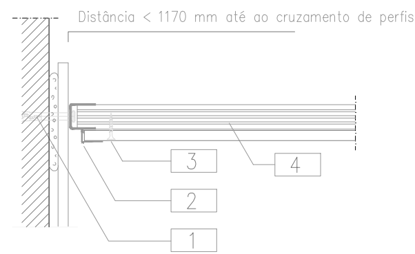
União entre muros: junta à vista
