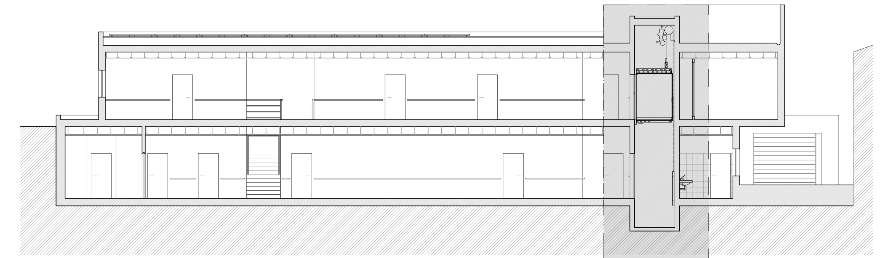
CORTE F-F PROPOSTO
