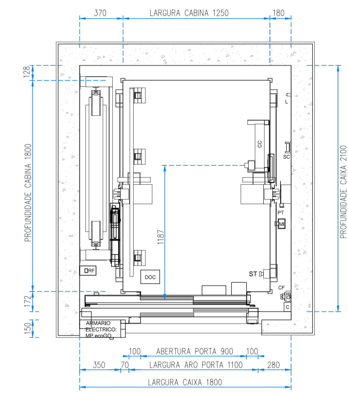
PLANTA Esc:1/20
