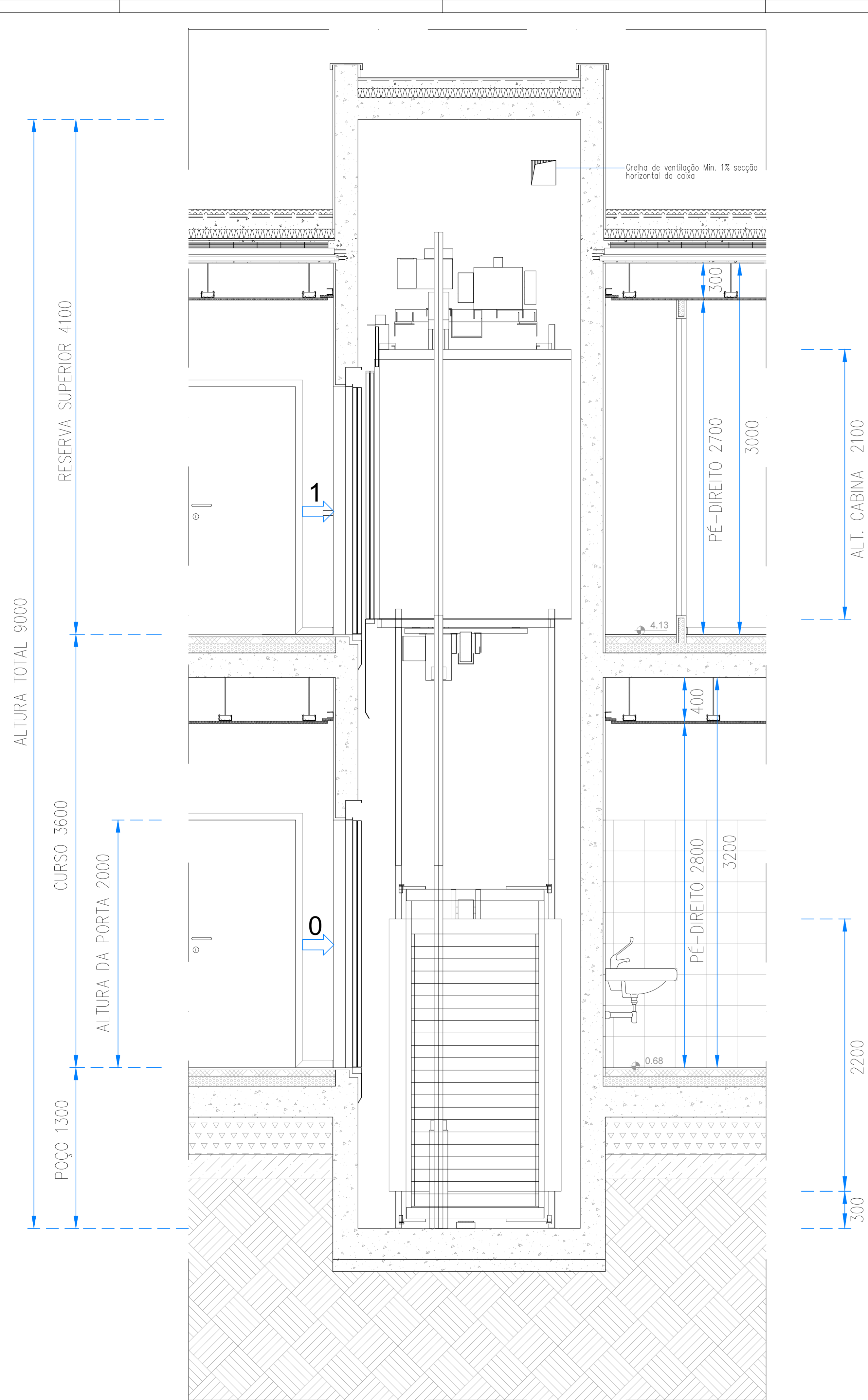
PORMENOR 6 Esc:1/20
