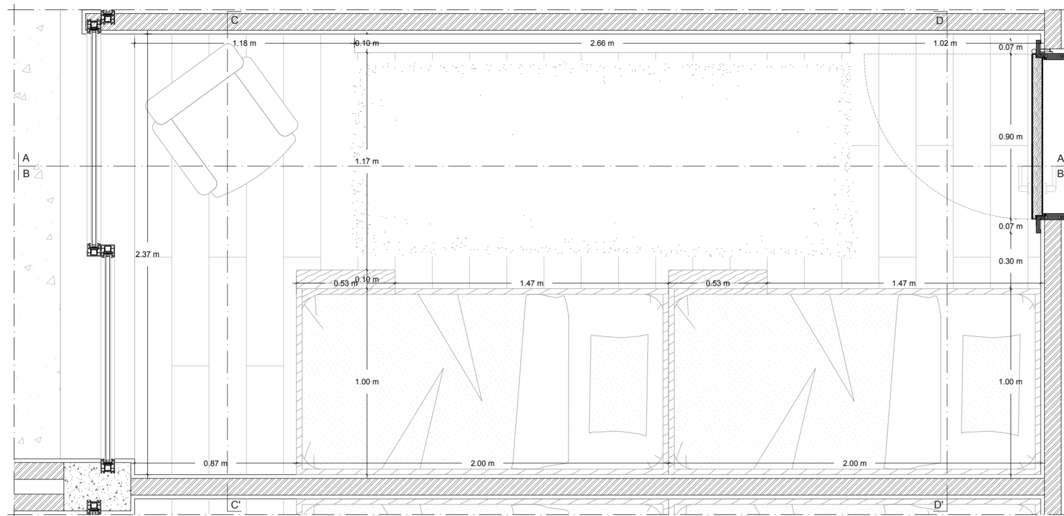
Planta pavimento
