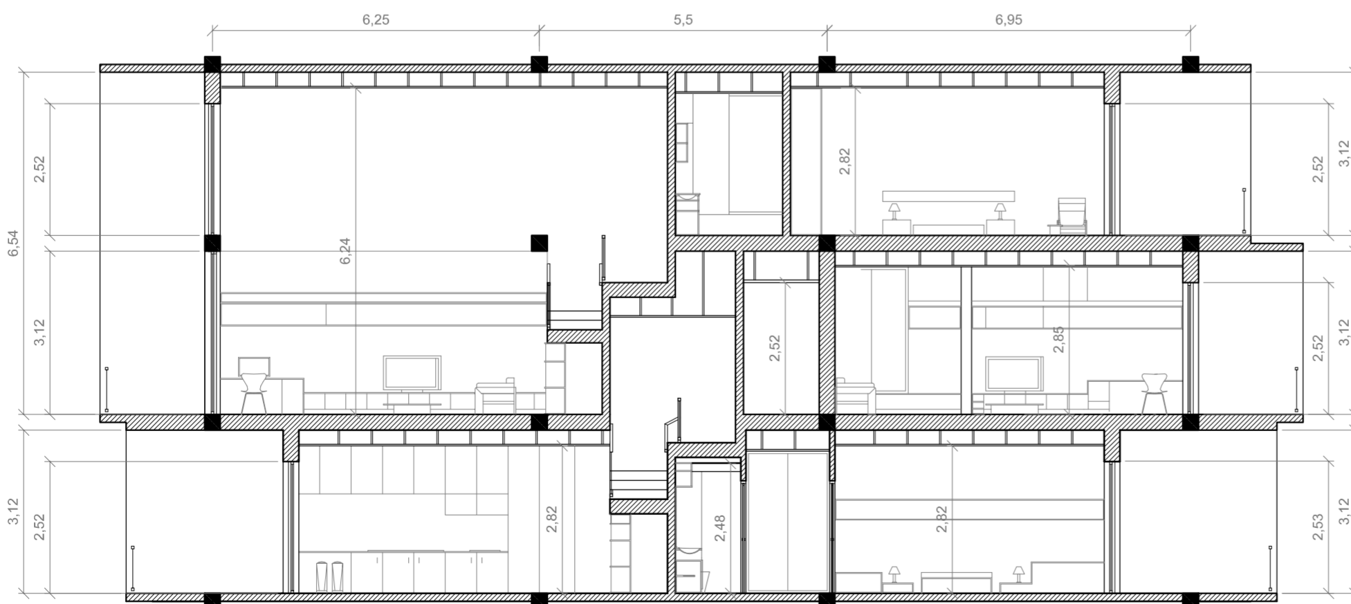
Corte AA'
