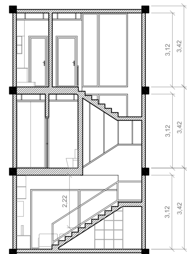
Corte BB'
