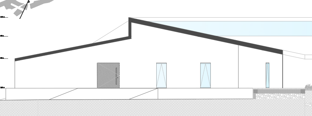
ALÇADO DO EDIFÍCIO DAS URGÊNCIAS VETERINÁRIAS
