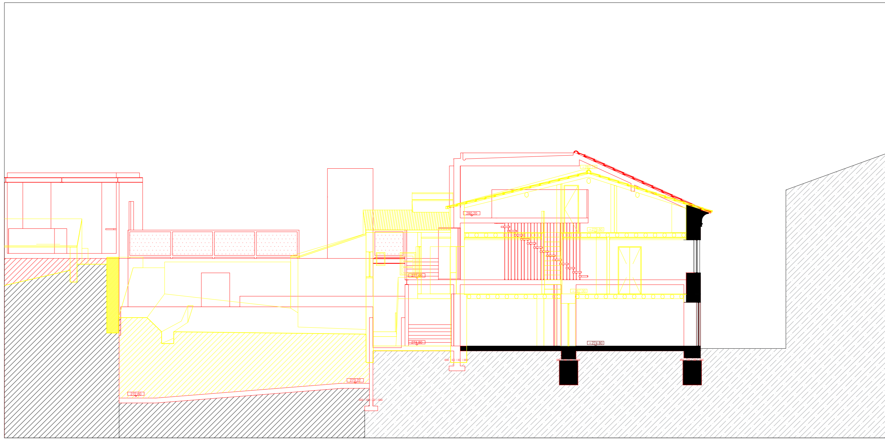
CORTE S3 ANEXO CASA PINA FALCÃO V.A
