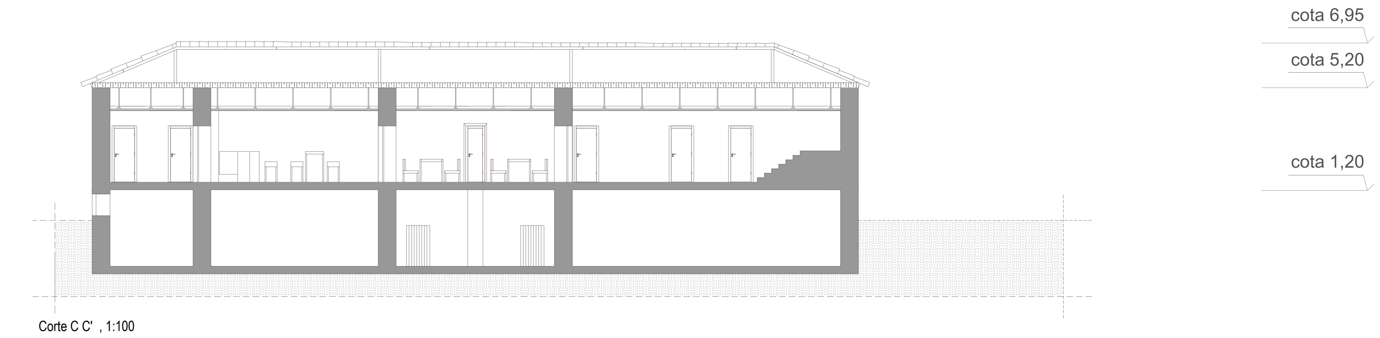
Corte C C', 1:100
