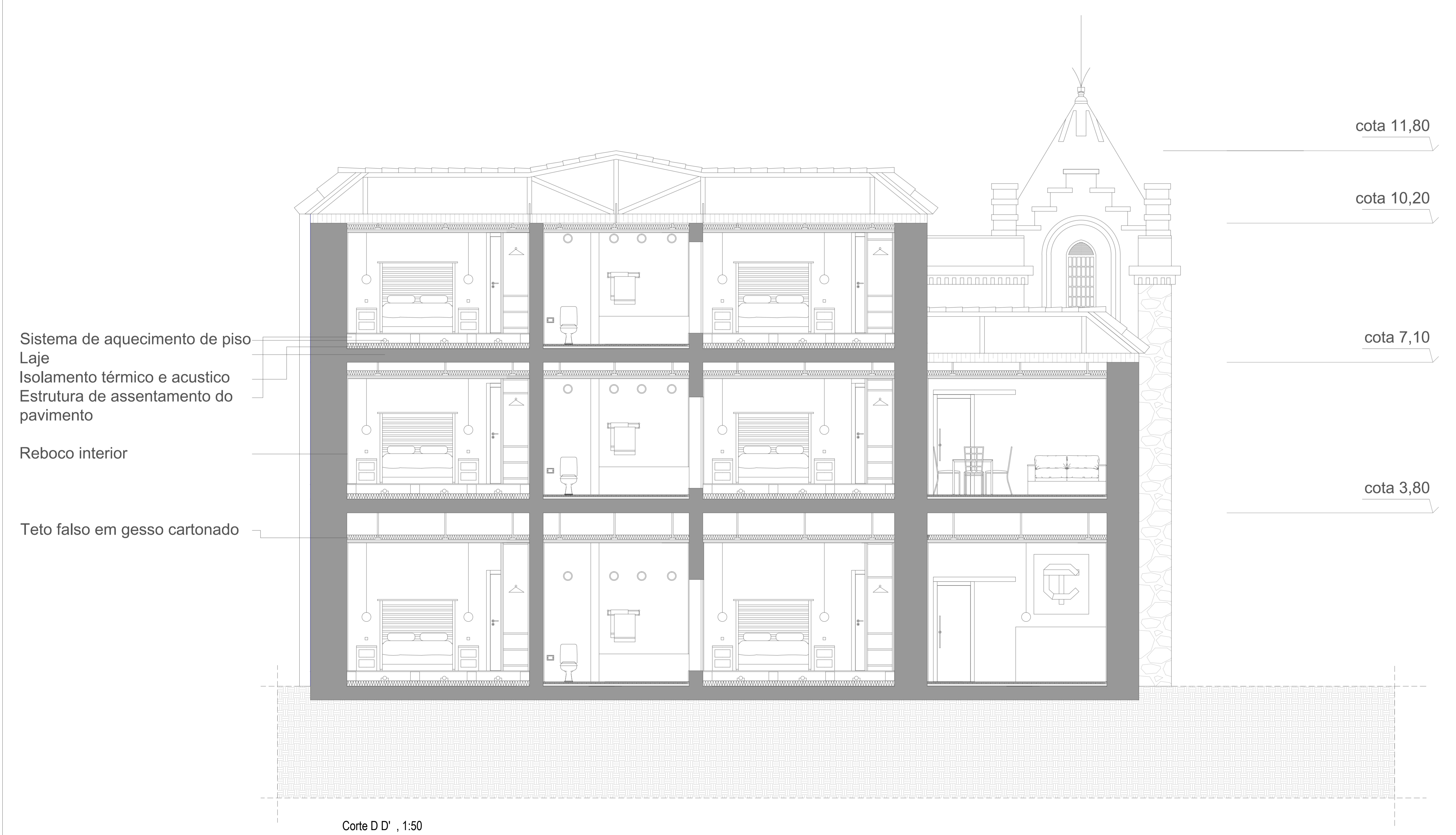
Corte D D', 1:50
