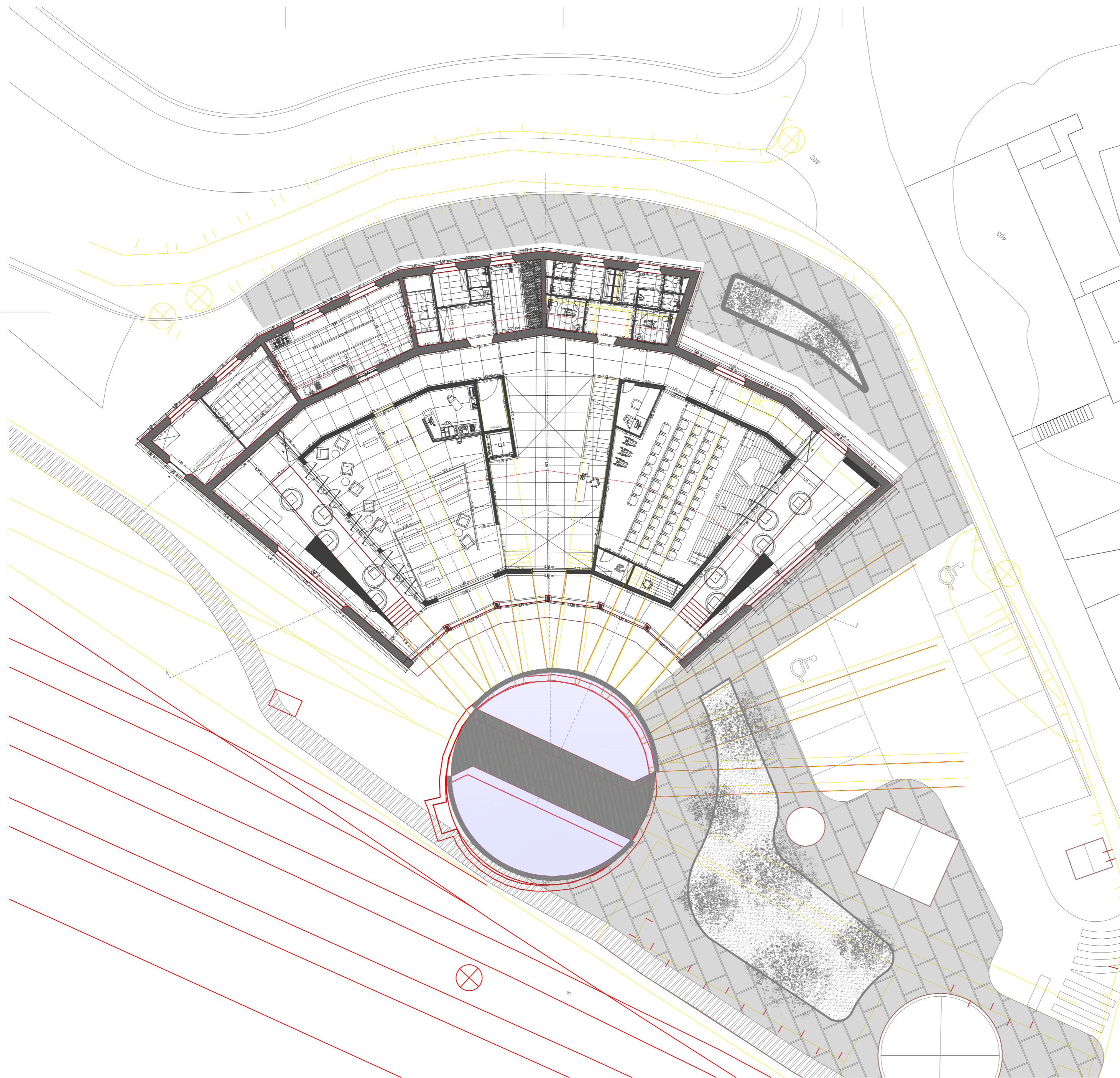
PLANTA DO PISO TÉRREO DO EDIFÍCIO DAS COCHEIRAS DOS COMBOIOS PROPOSTA E VERMELHOS E AMARELOS
