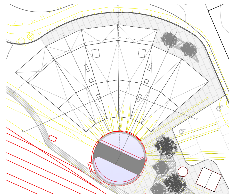
PLANTA DE COBERTURA DO EDIFÍCIO DAS COCHEIRAS DOS COMBOIOS PROPOSTA E VERMELHOS E AMARELOS
