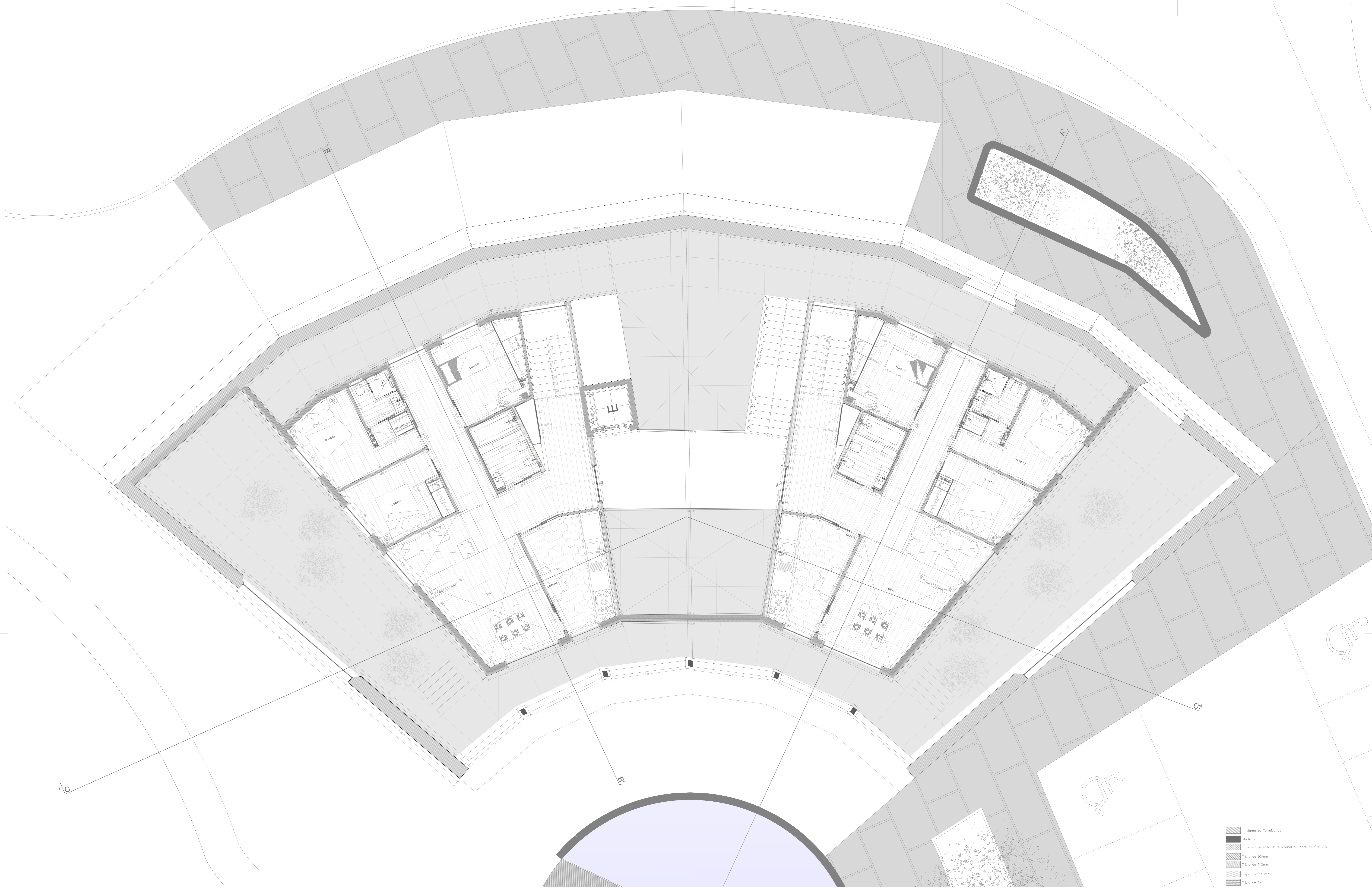
PLANTA PISO 1 DO EDIFÍCIO DAS COCHEIRAS DOS COMBOIOS
