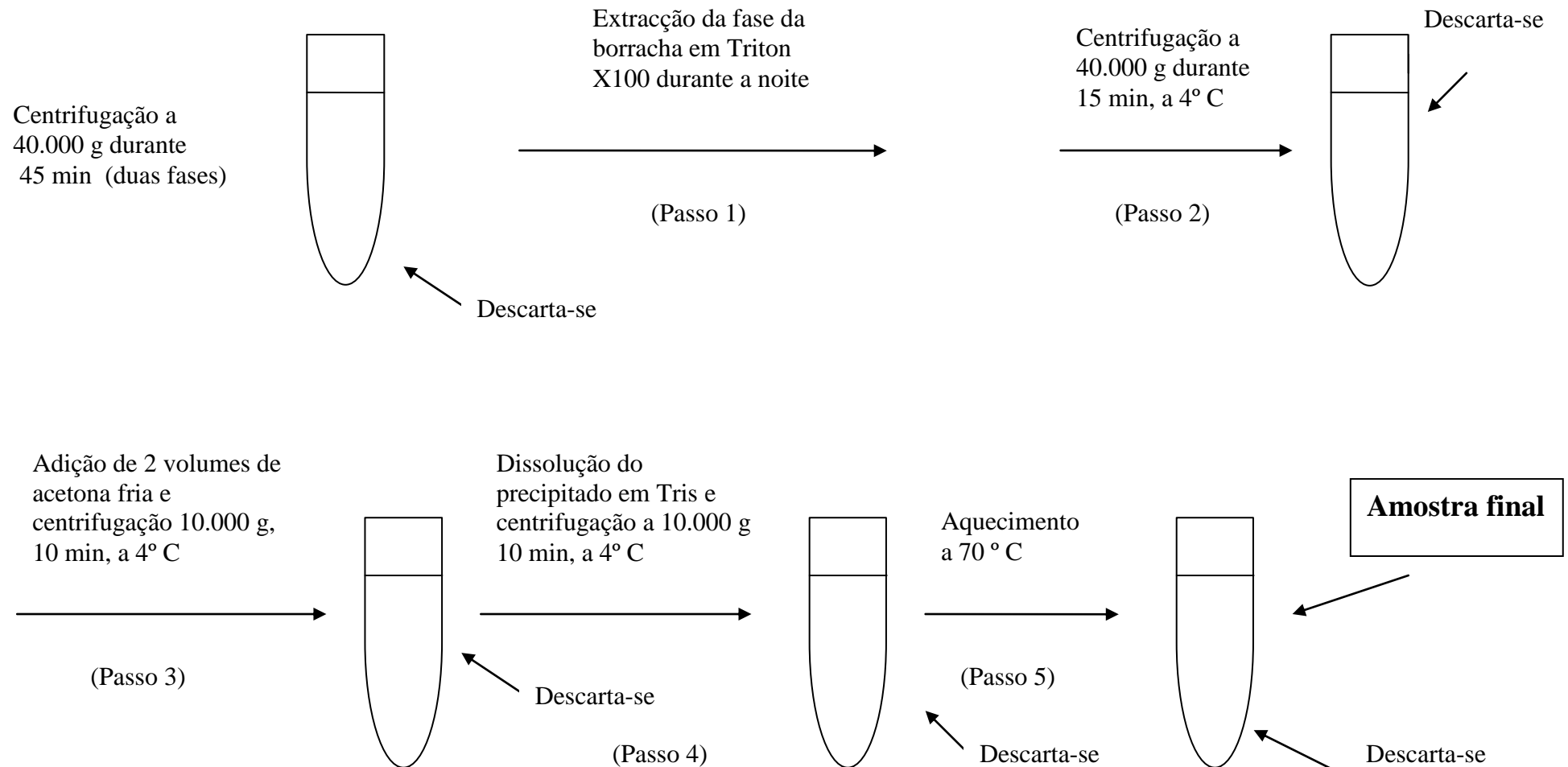
Figura 4.2: Esquema que representa os diversos passos de extracção pelo método de Wititsuwannakul (Wititsuwannakul et al. , 2008)
