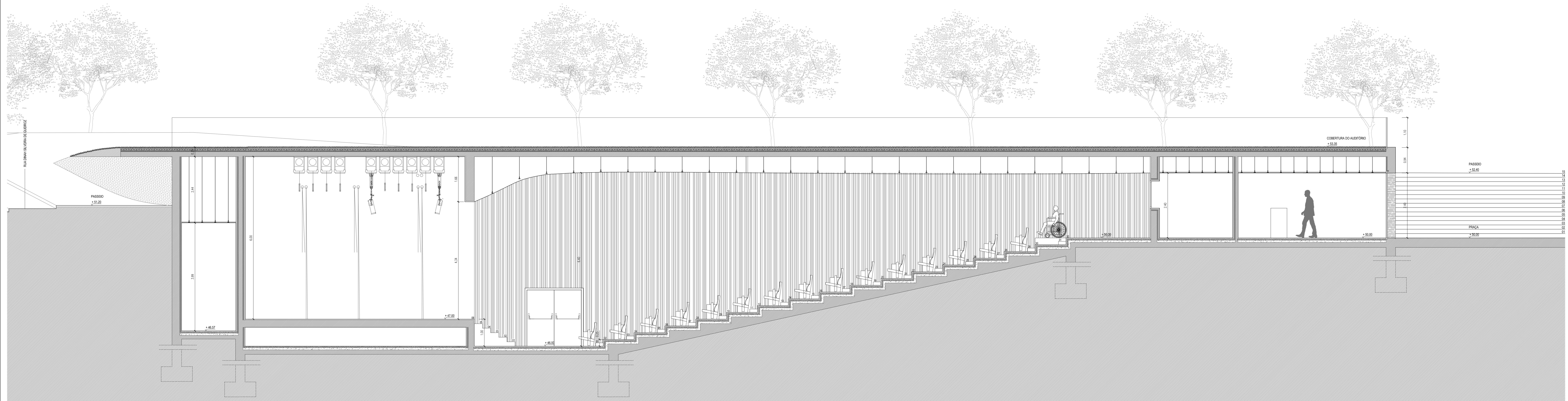
CORTE LONGITUDINAL 3 - PARTE II AUDITÓRIO
