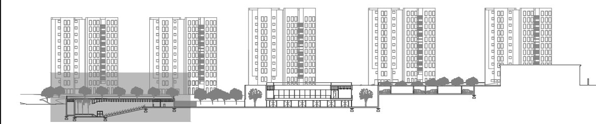
CORTE LONGITUDINAL 3 - PARTE II AUDITÓRIO
