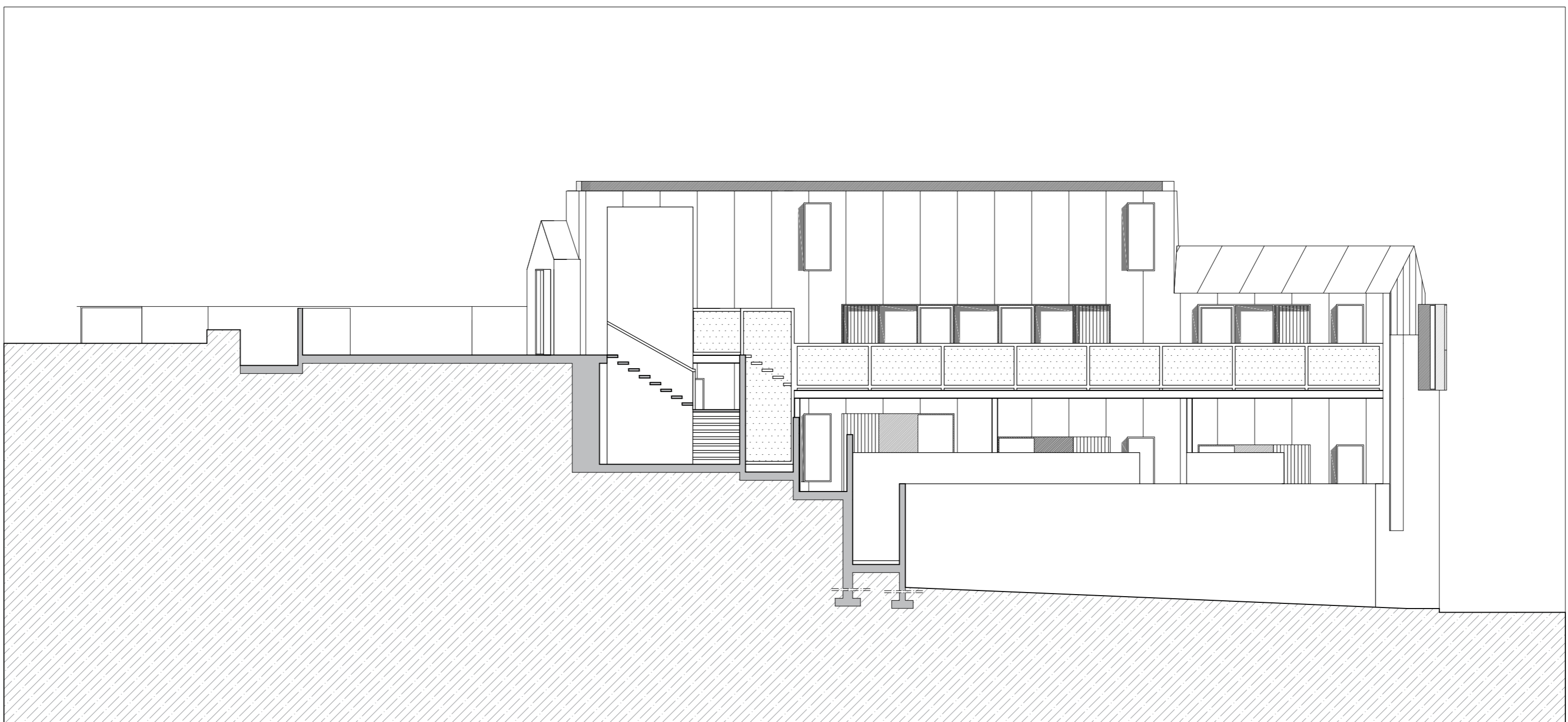
CORTE O4 ANEXOS CASA PINA FALCÃO
