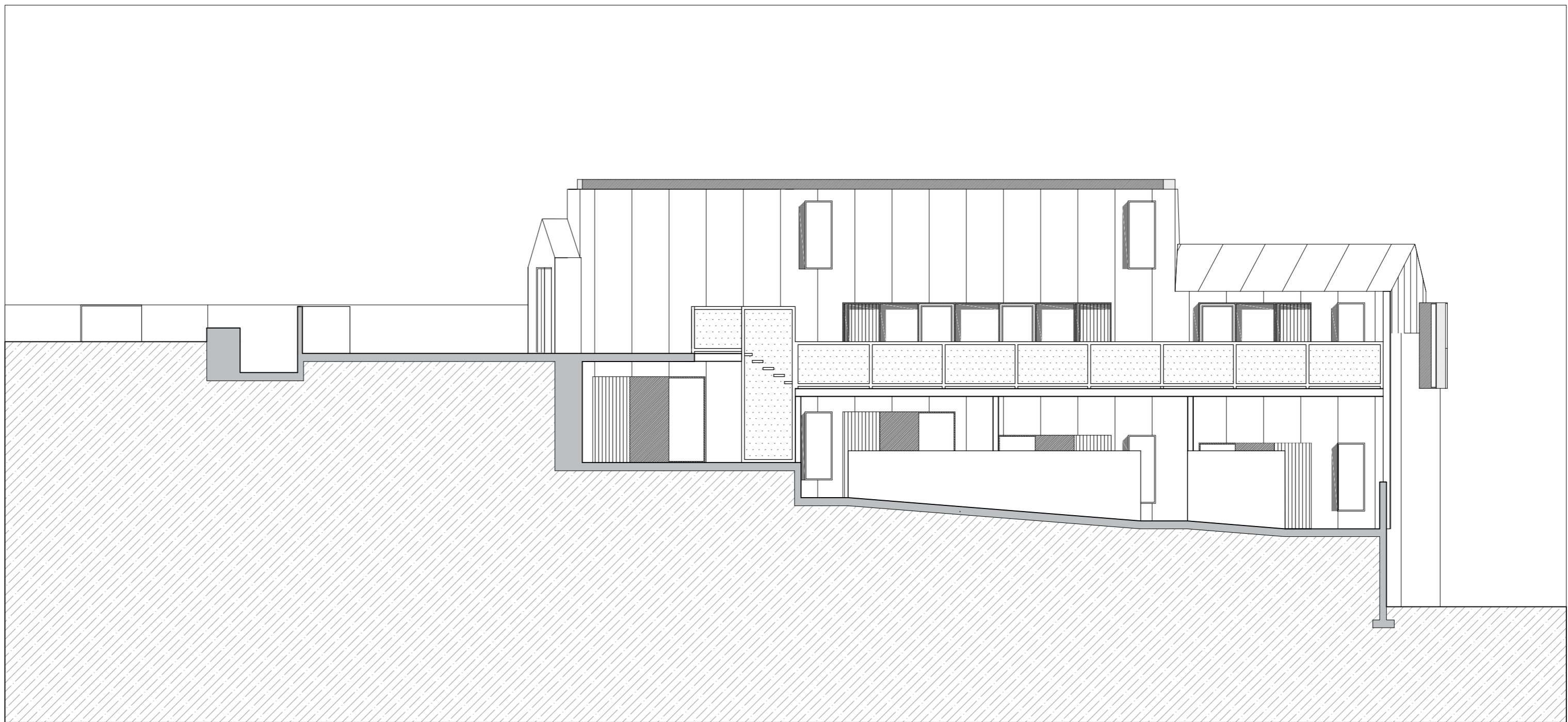
CORTE O3 ANEXOS CASA PINA FALCÃO
