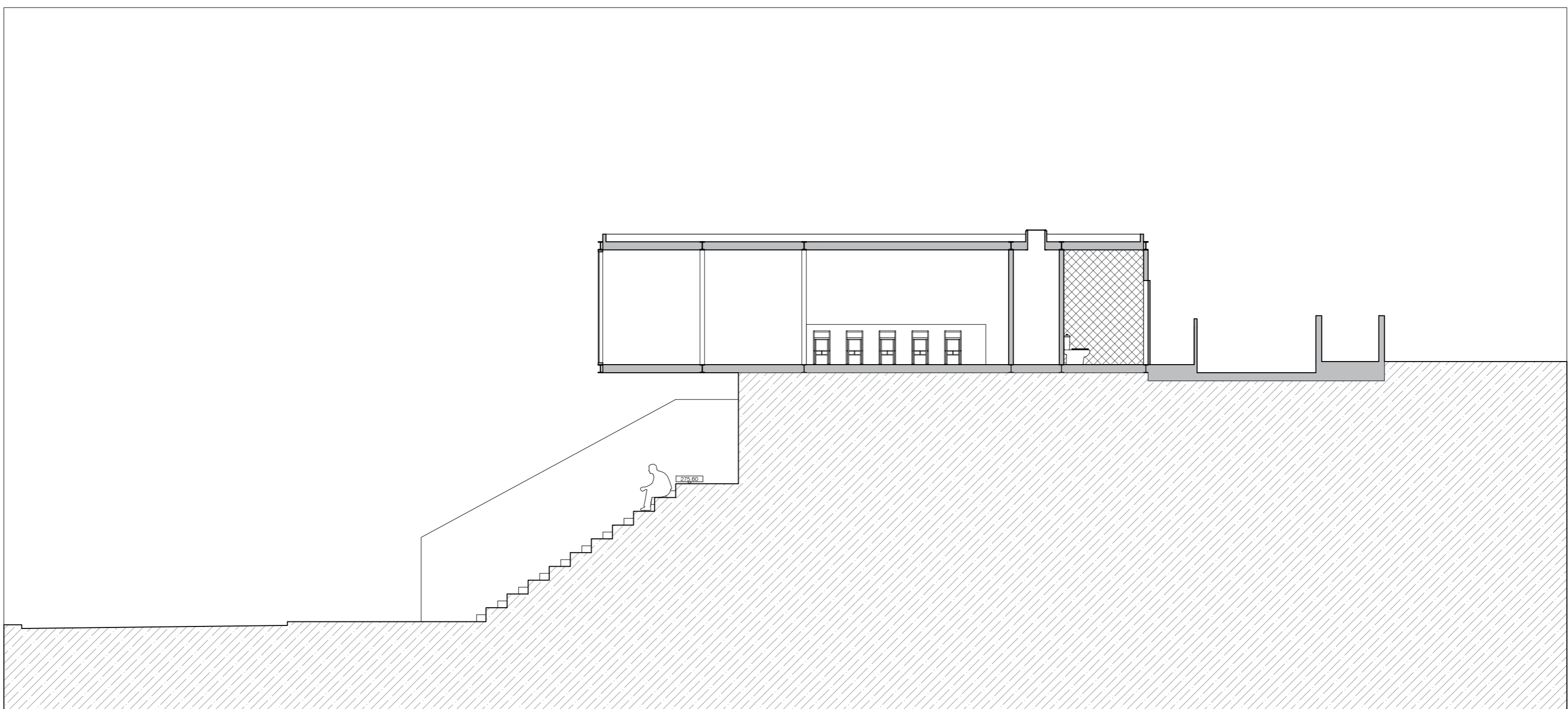
CORTE E1 ANEXOS CASA PINA FALCÃO
