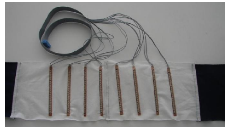
Fig. 3. Flex sensor belt.
