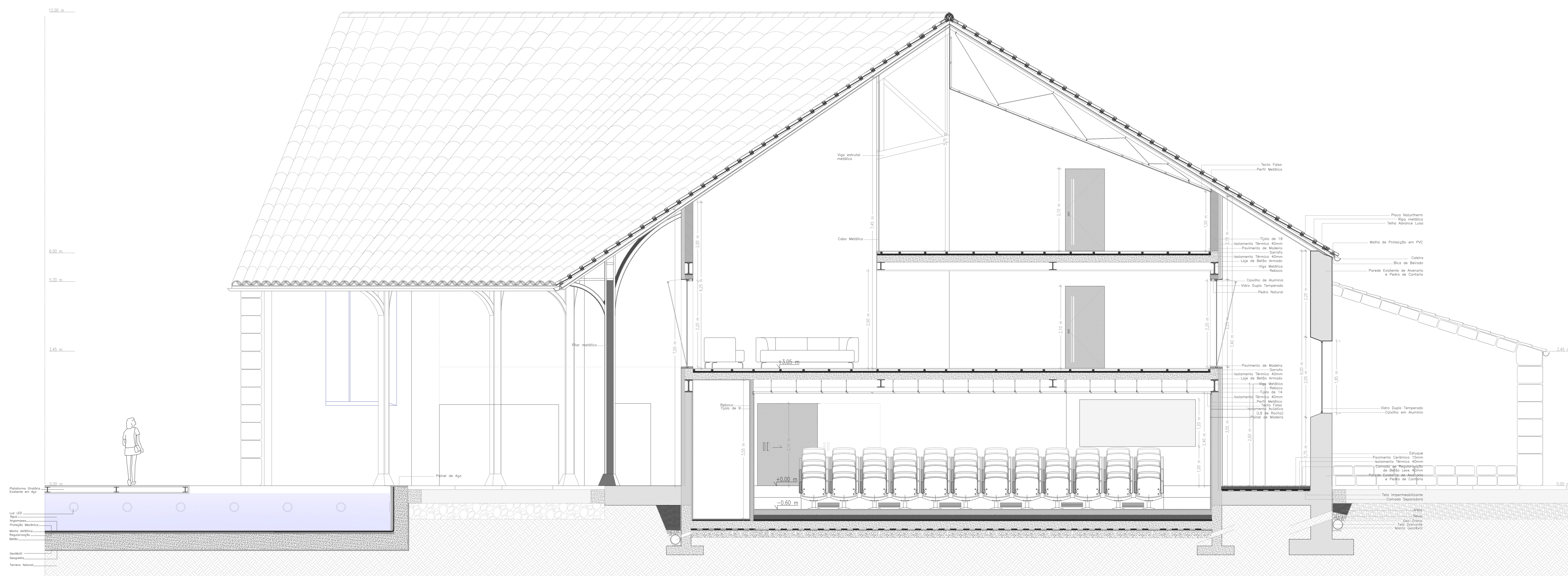
Corte AA'
