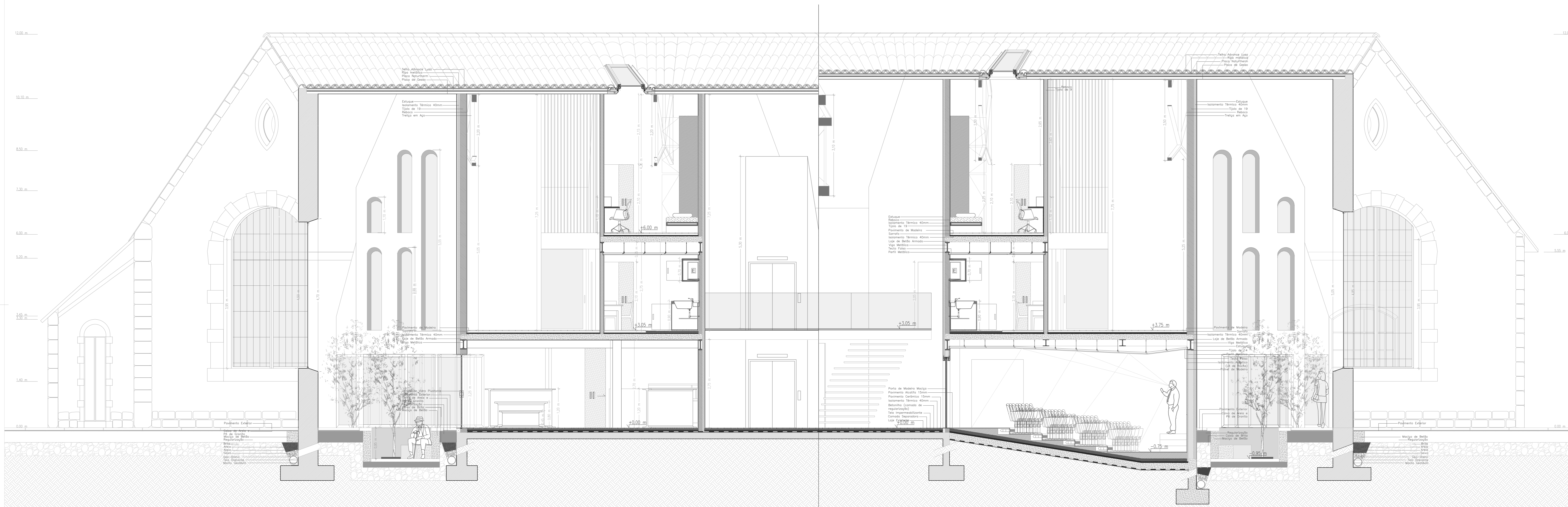
Corte CC'
