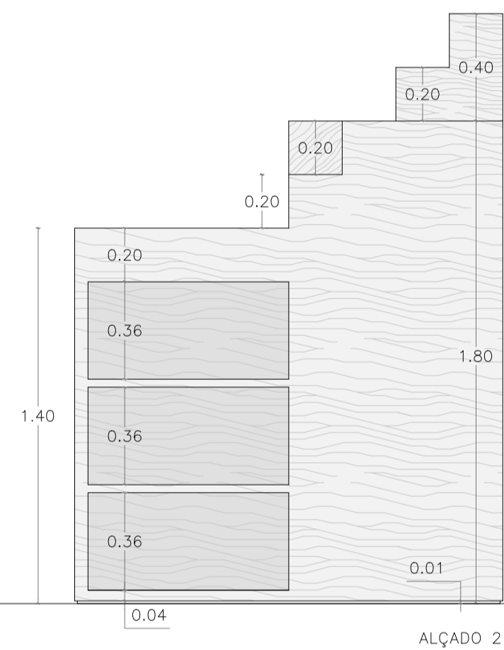
ALÇADO 2
