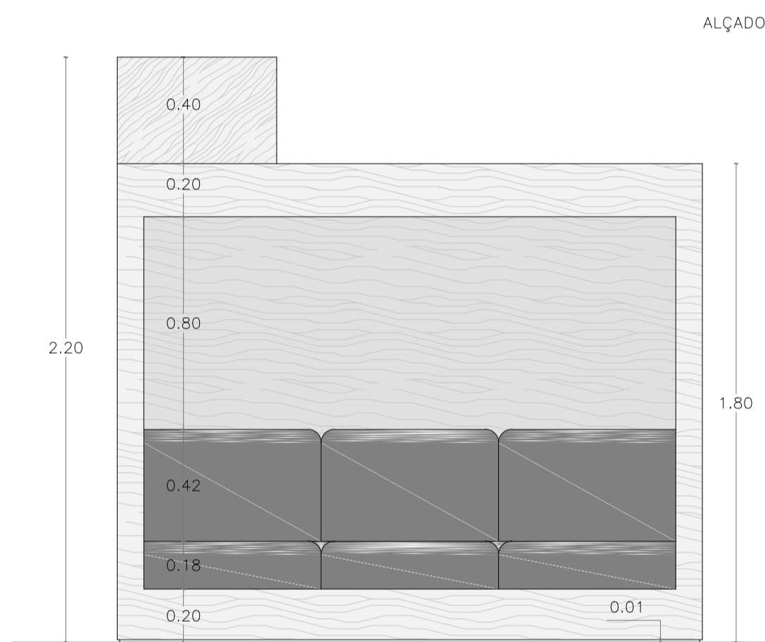
ALÇADO 1
