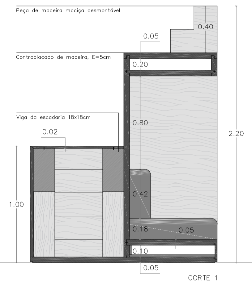
CORTE 1
