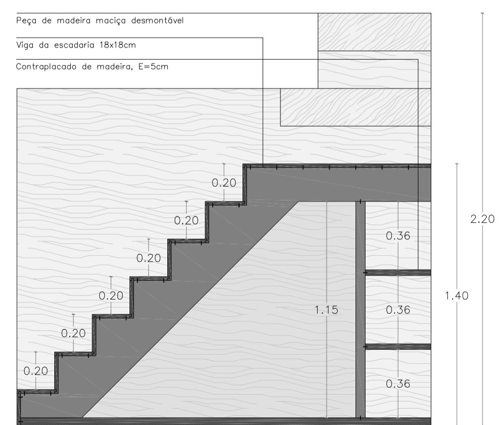
CORTE 2
