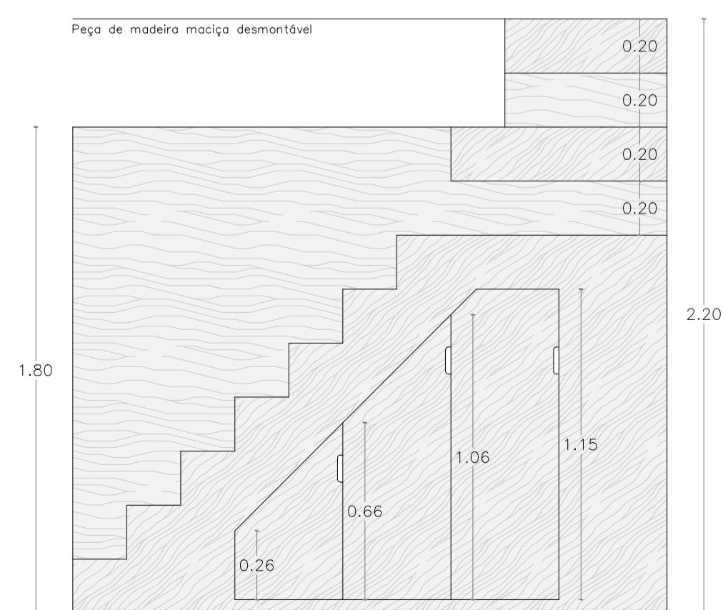
ALÇADO 4
