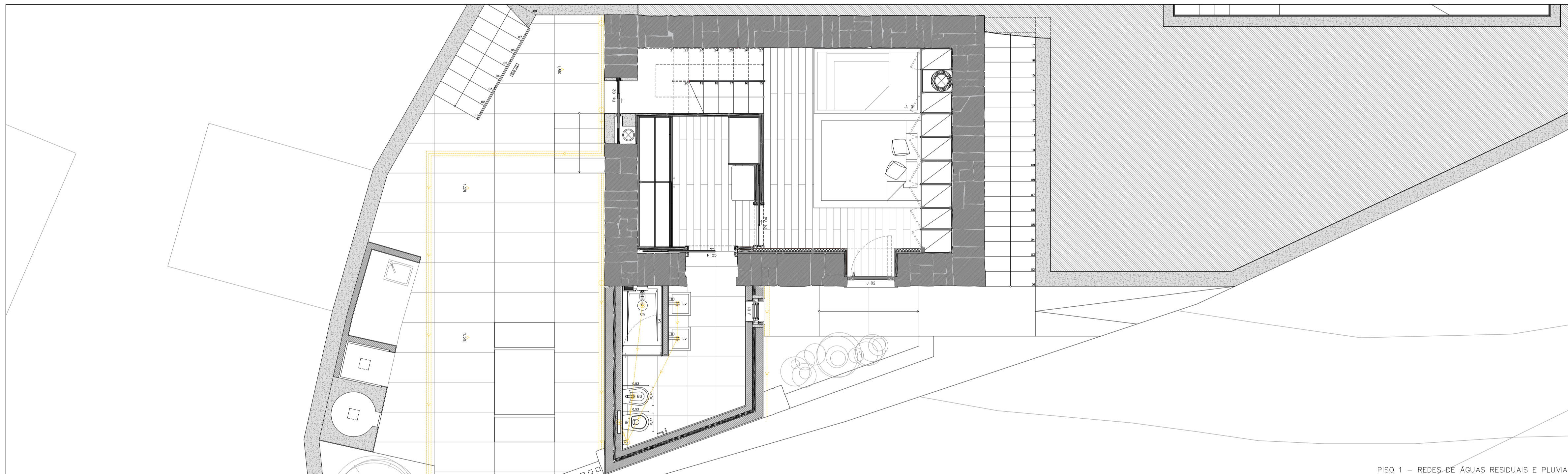
PISO 1 – REDES DE ÁGUAS RESIDUAIS E PLUVIAIS
