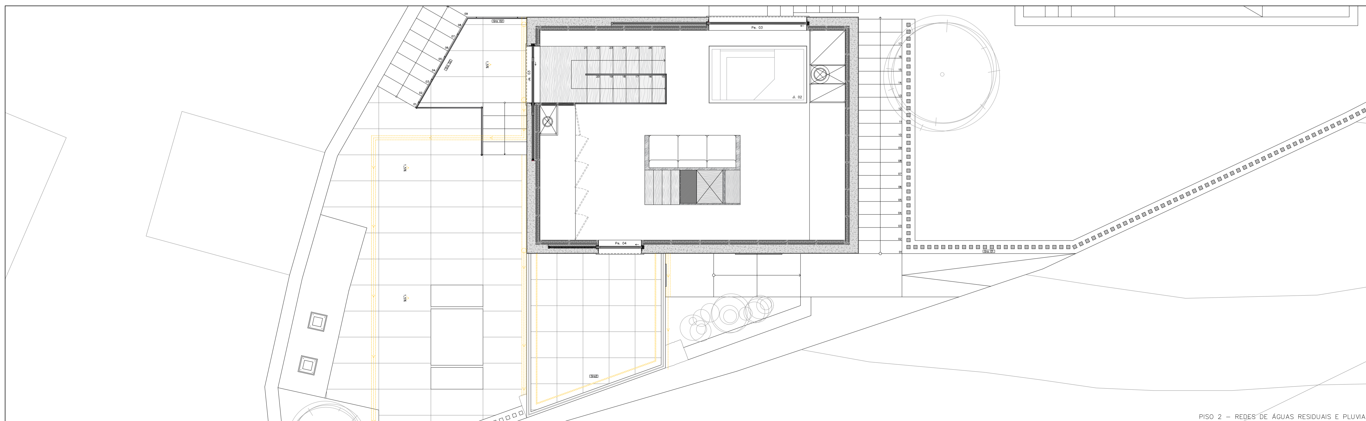
PISO 2 – REDES DE ÁGUAS RESIDUAIS E PLUVIAIS
