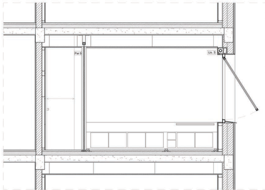
Corte EE'
