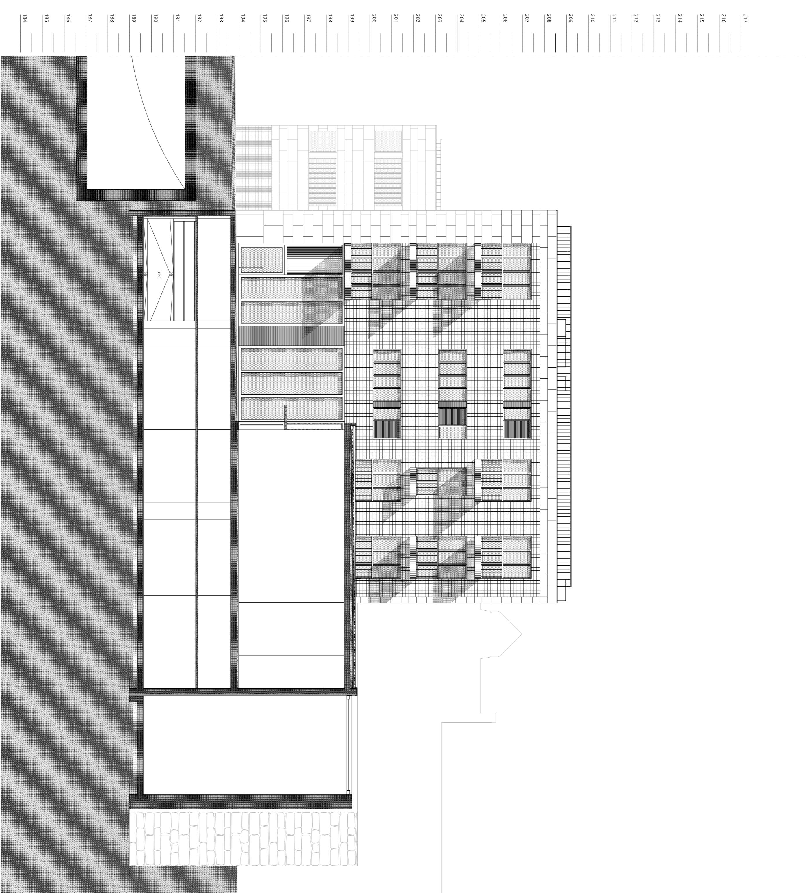
EDIFÍCIO B - alçado Nascente / corte DD.
