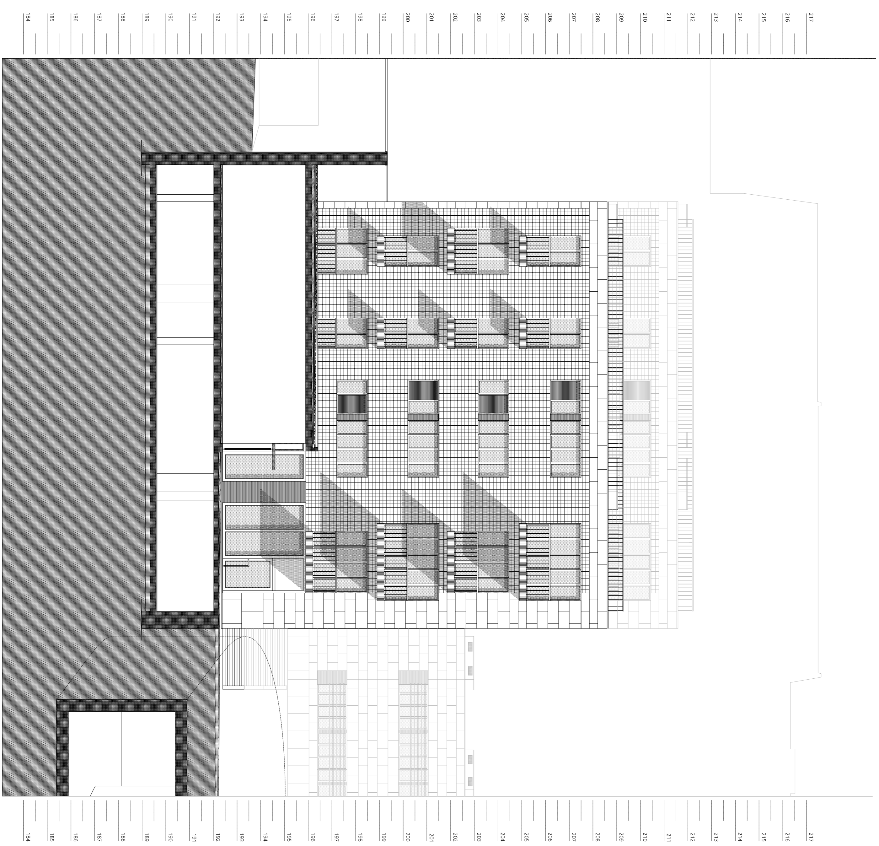
EDIFÍCIO B - alçado Poente / corte CC.
