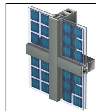
CÉLULAS FOTOVOLTAICAS 120X120 CM
