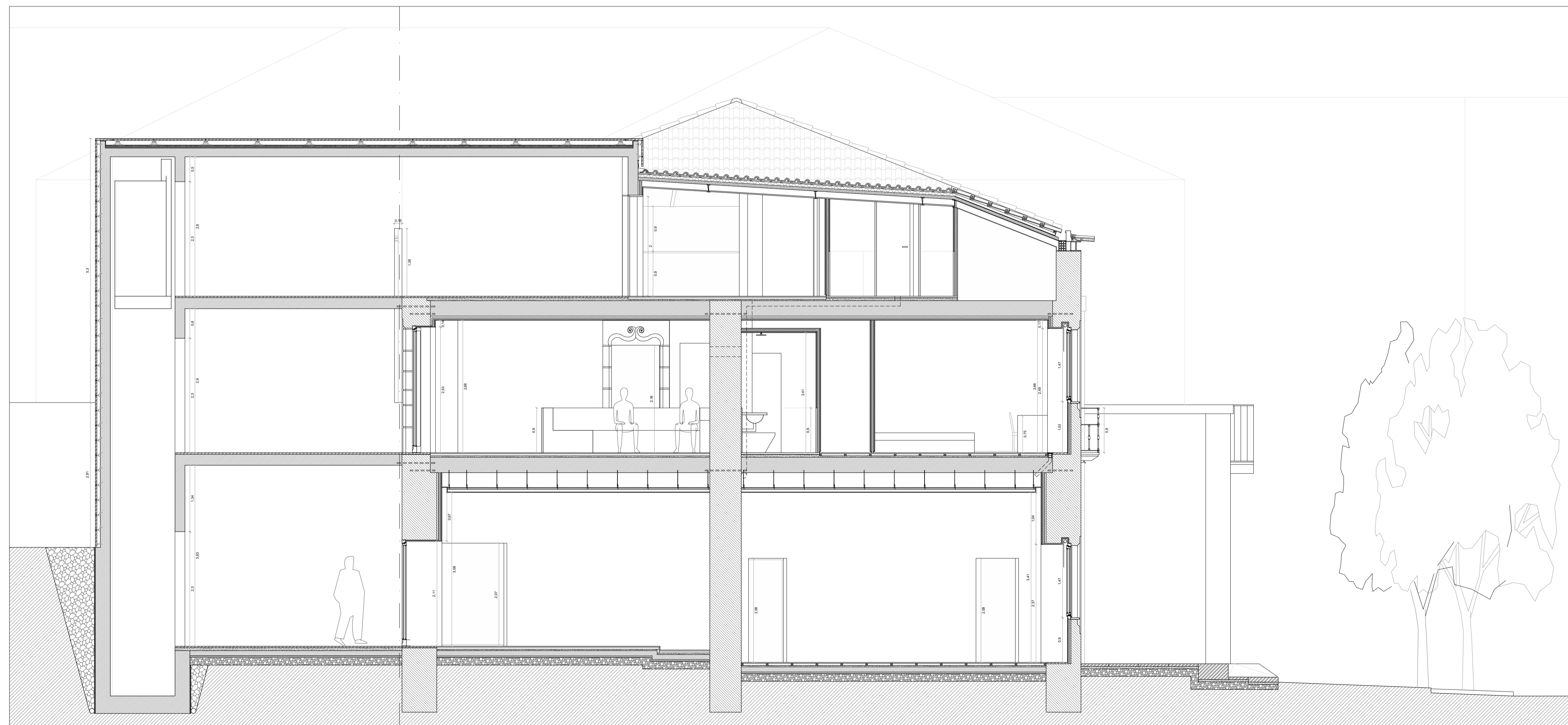
CORTE 2
