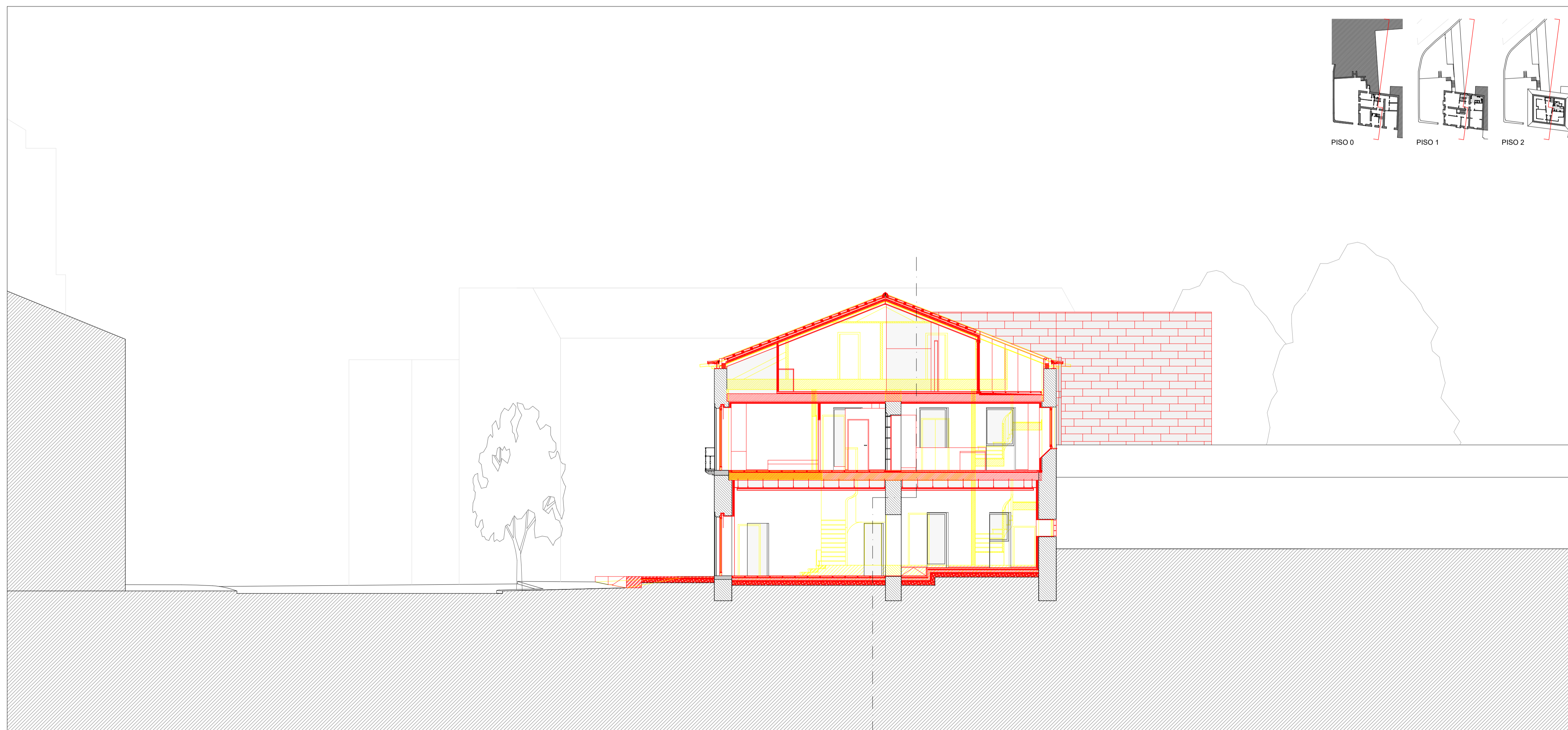
CORTE 02
