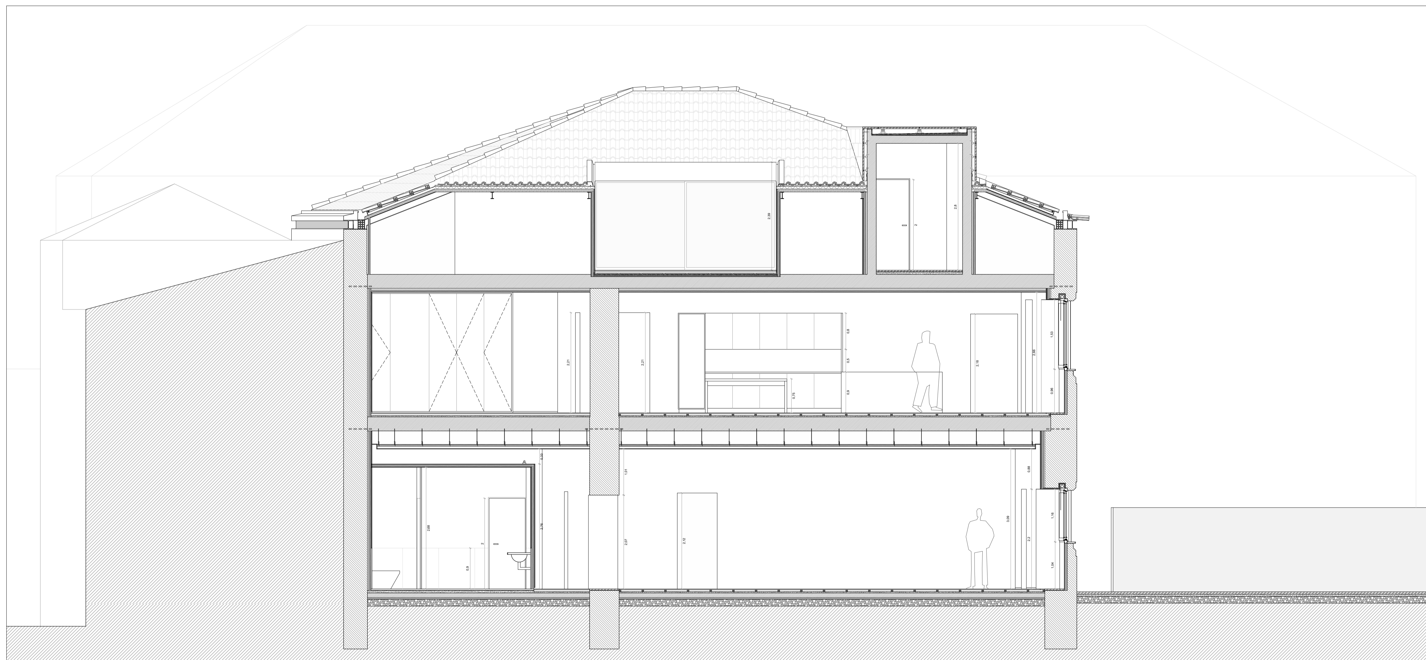
CORTE 4
