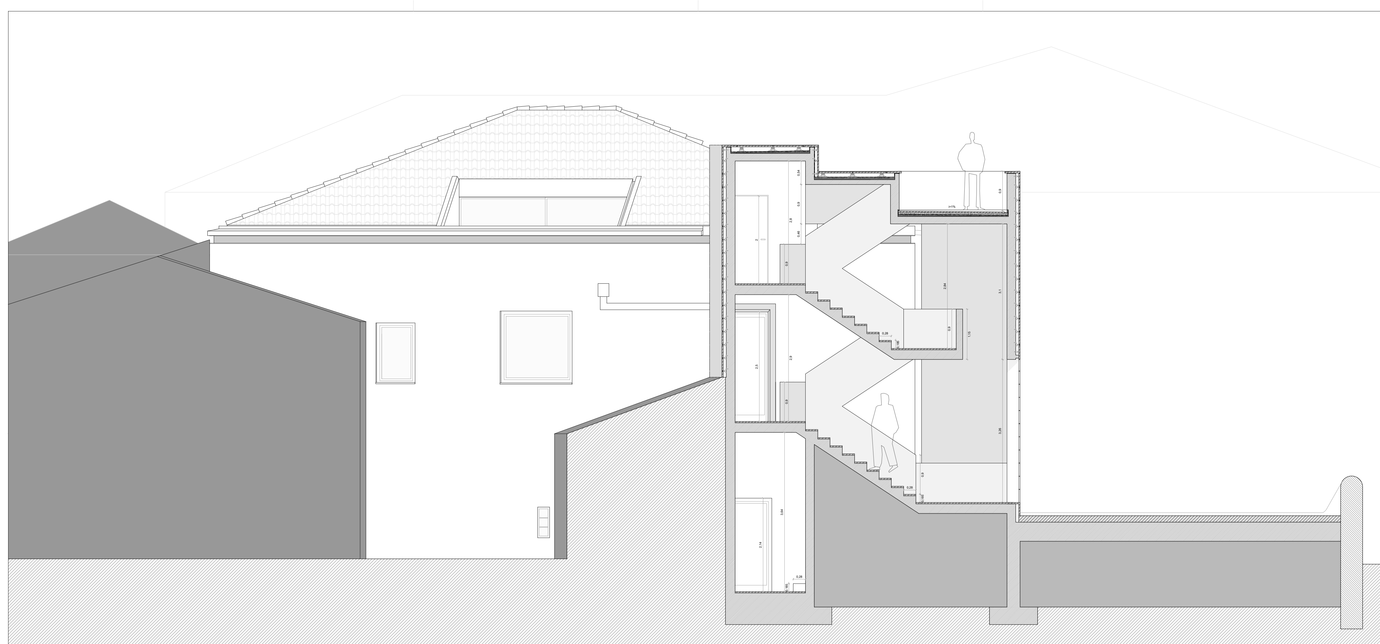
CORTE ALÇADO NORTE 5
