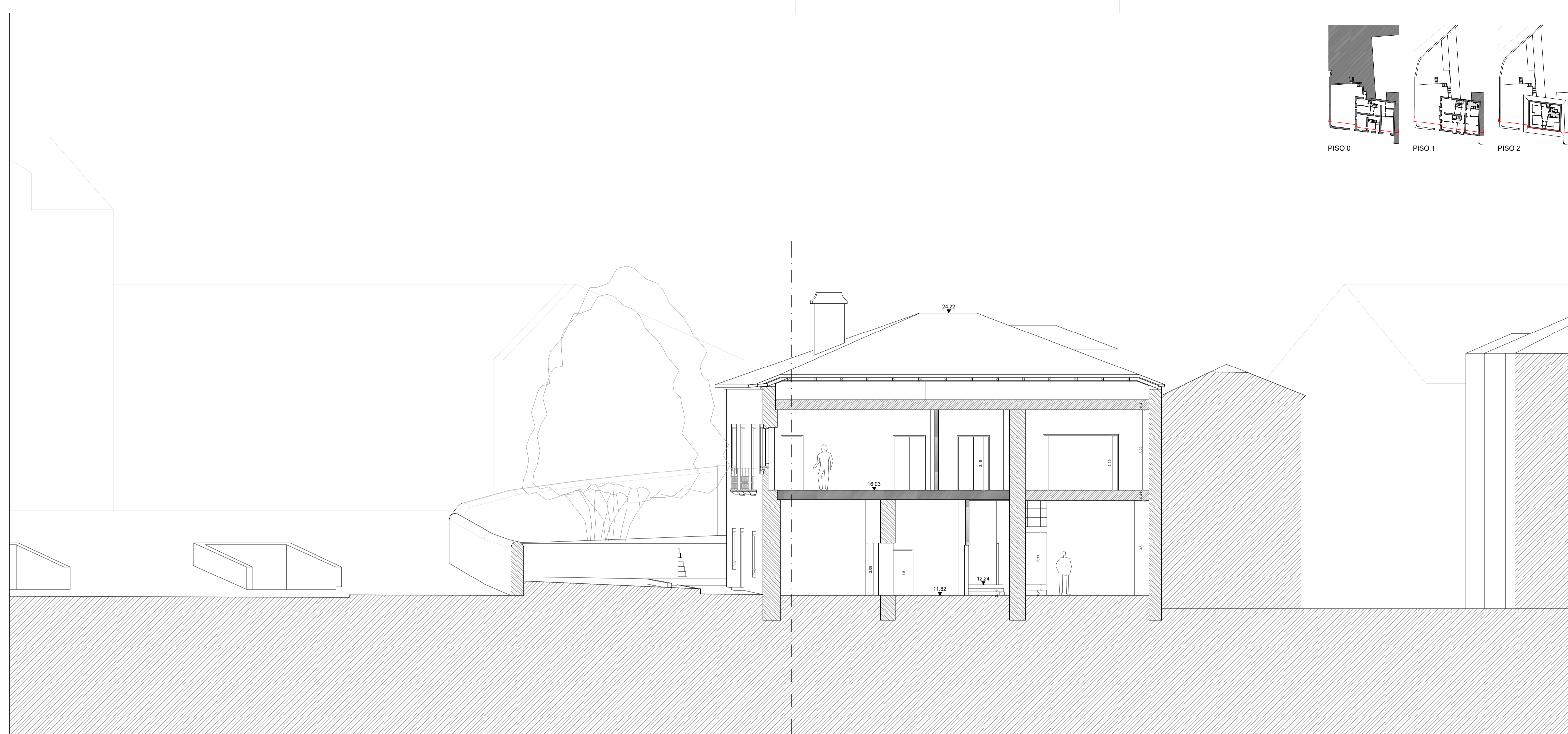
CORTE 03
