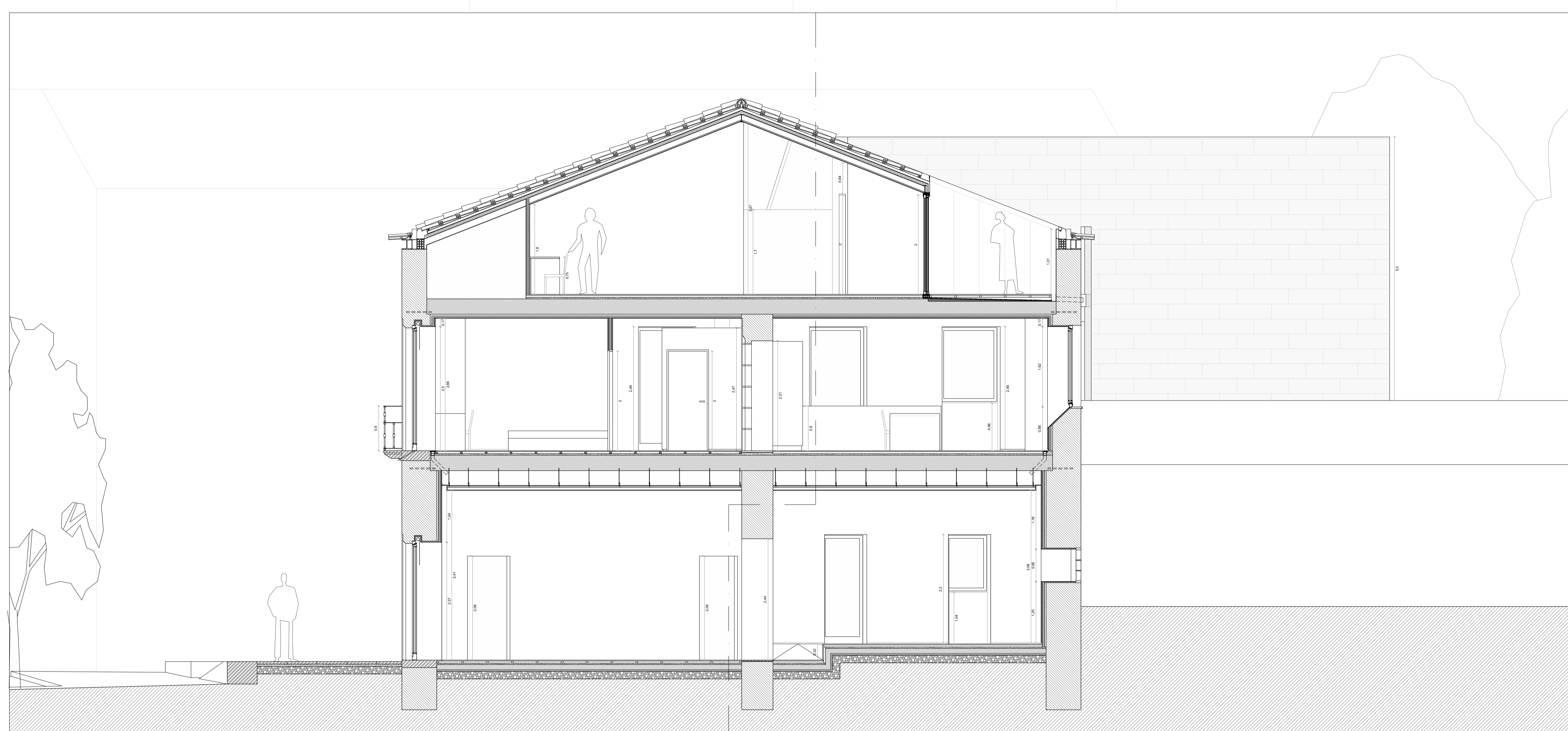
CORTE 1
