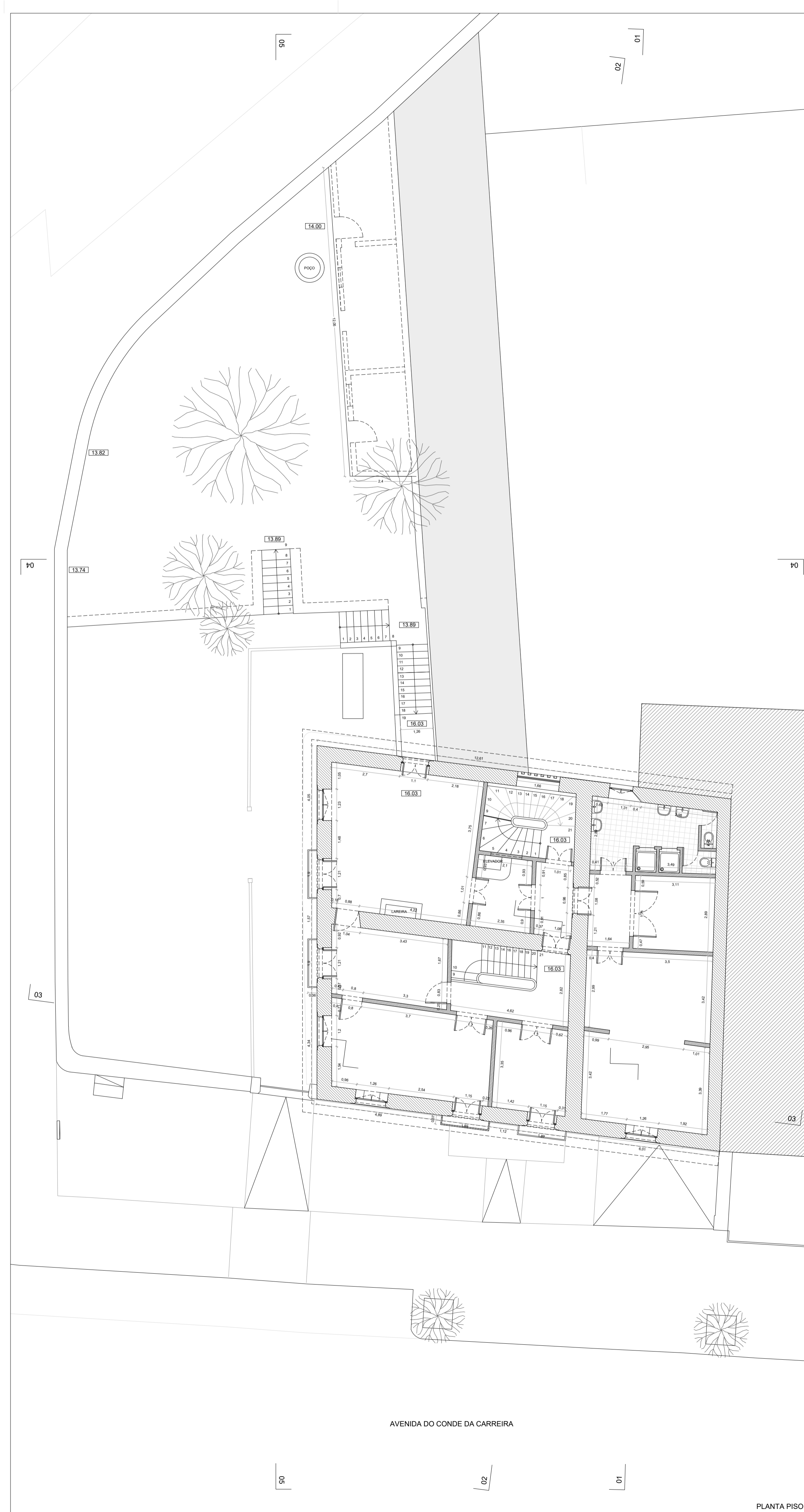
PLANTA PISO 1
