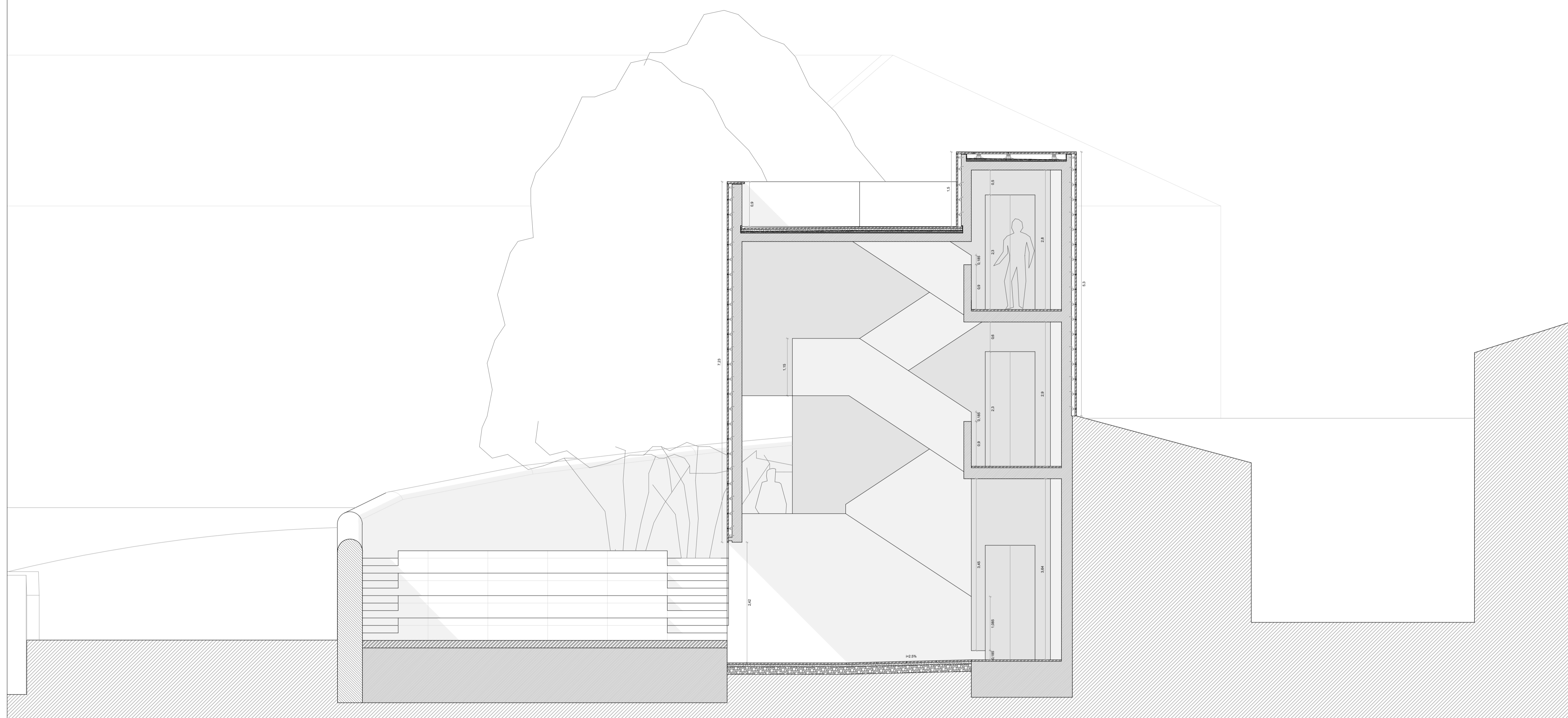
CORTE 3
