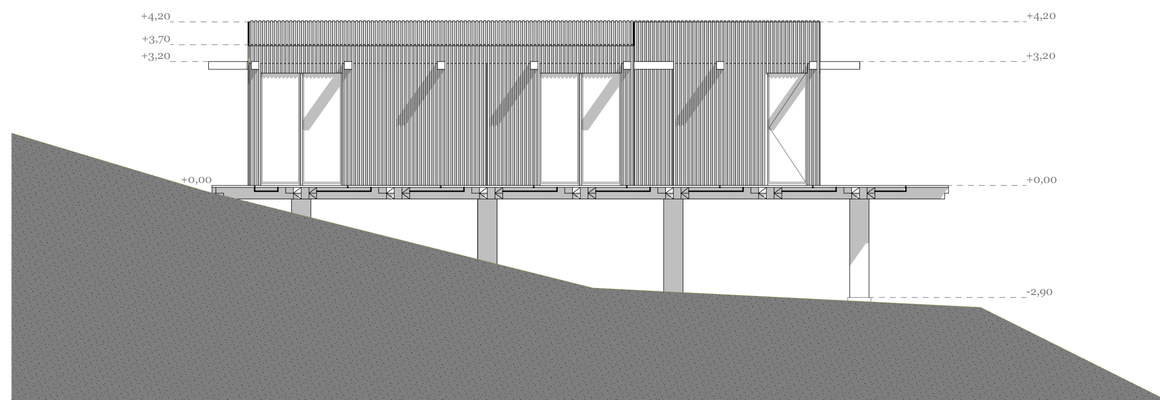
ALÇADO OESTE
