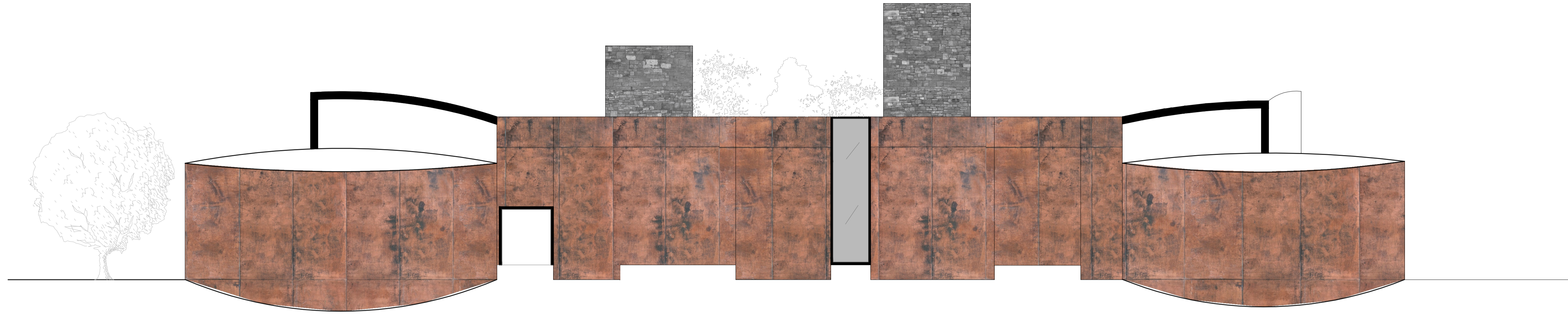
ALÇADO SUL
