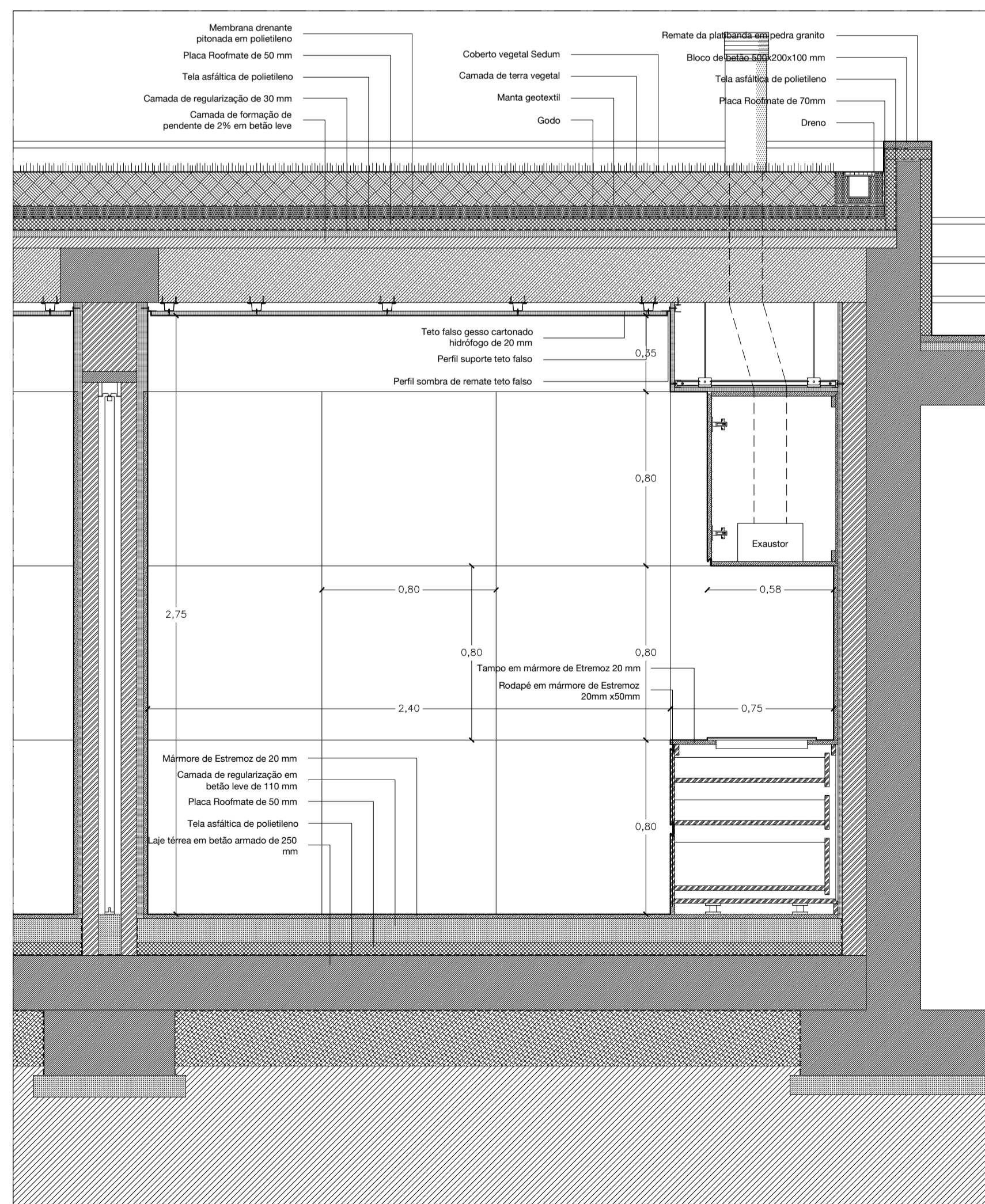
Corte d-d
