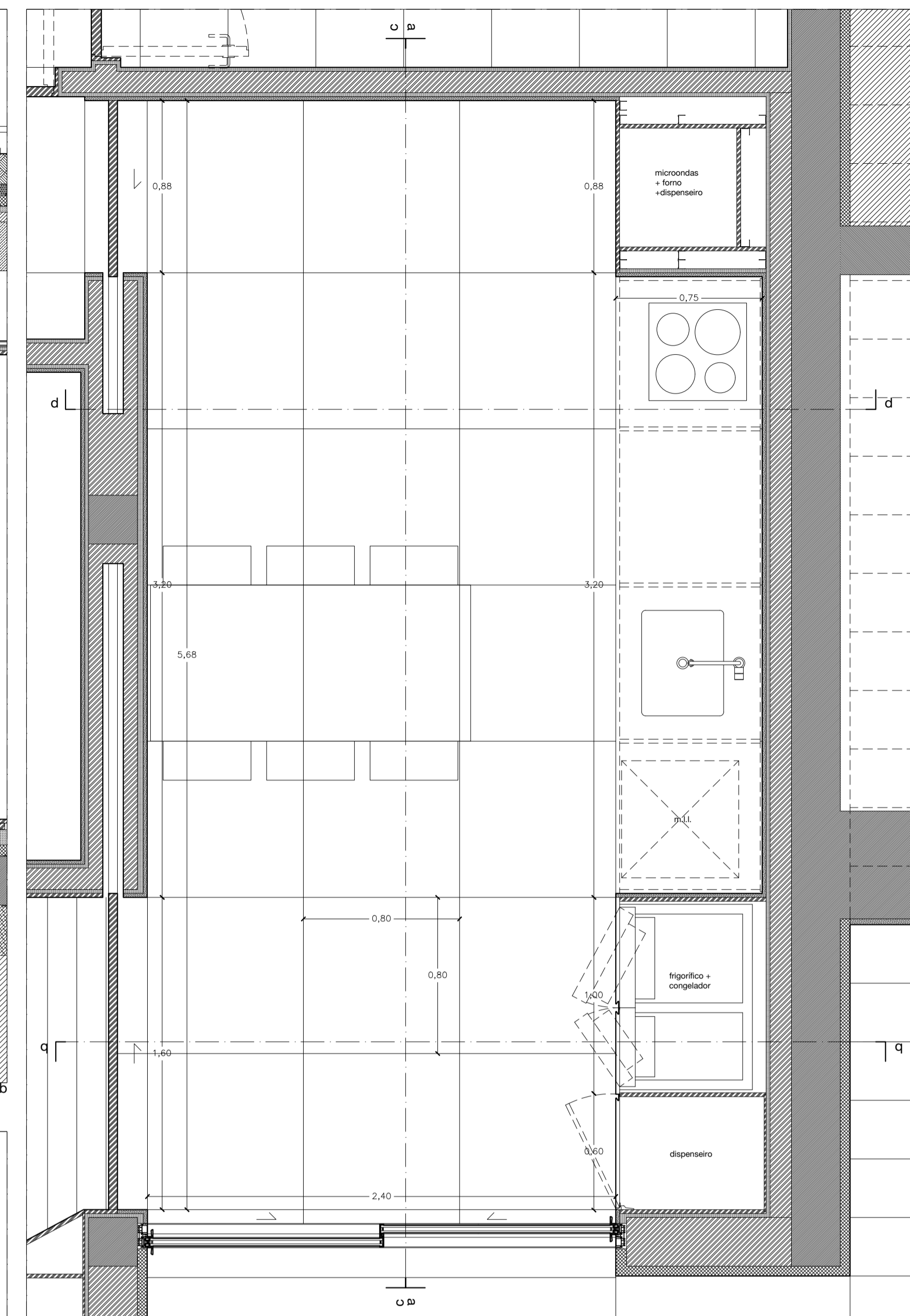
Planta
