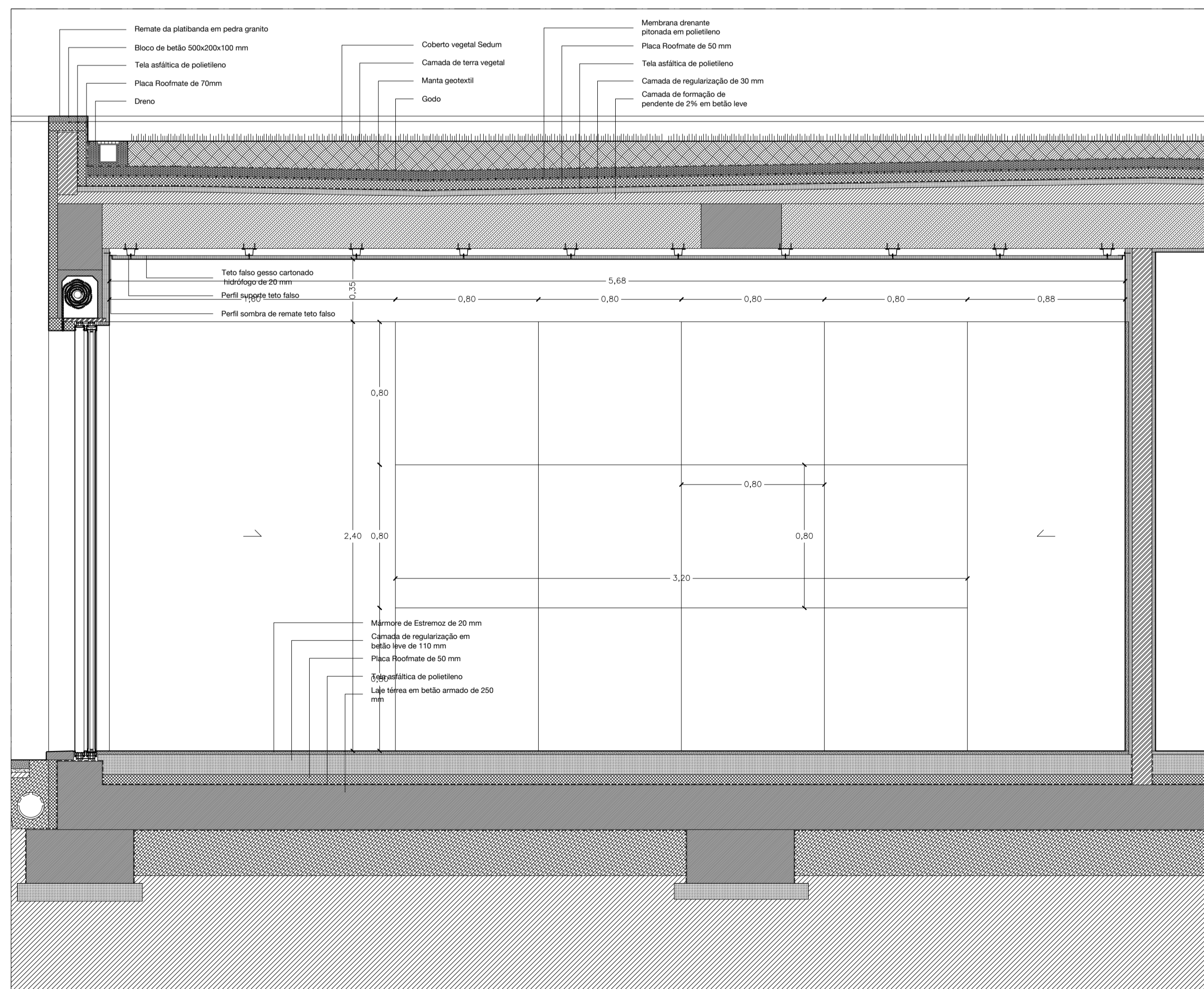
Corte c-c
