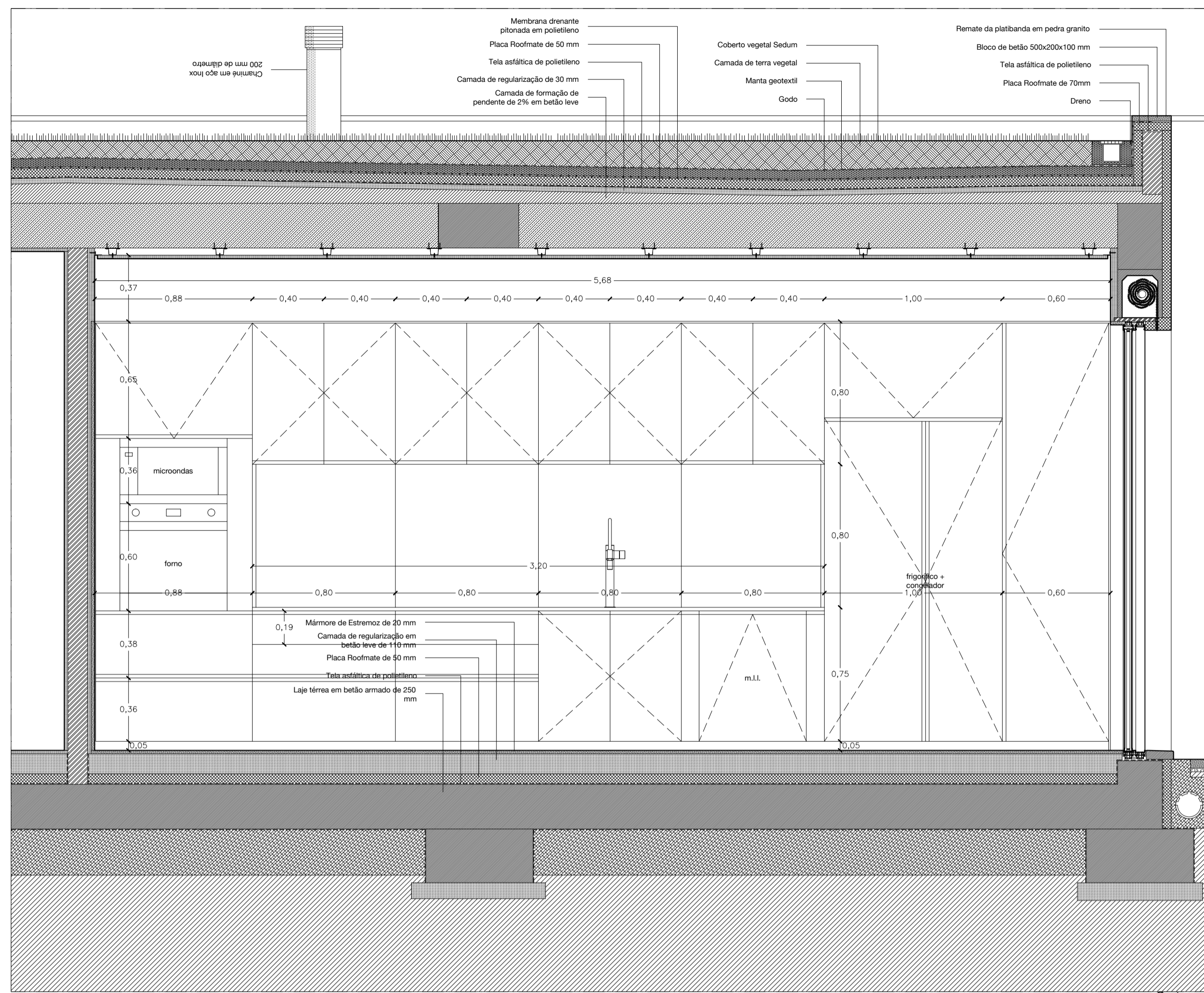
Corte a-a
