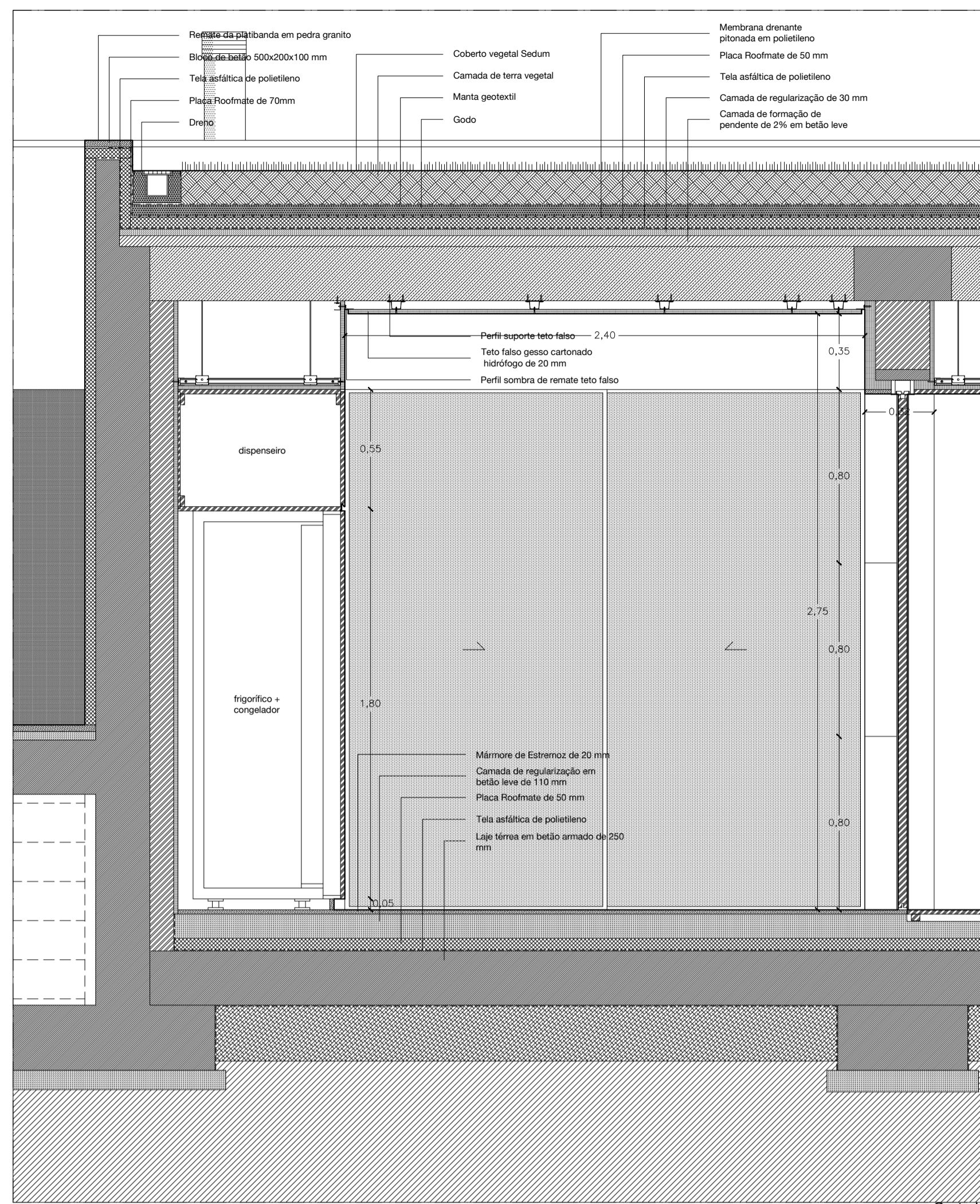
Corte b-b
