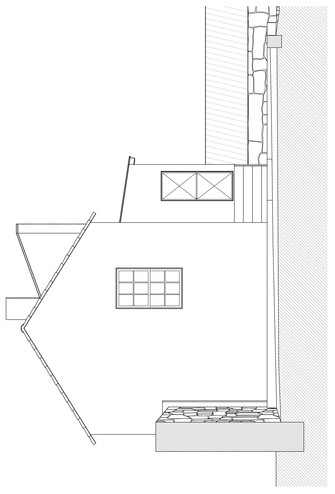
Alçado Norte
