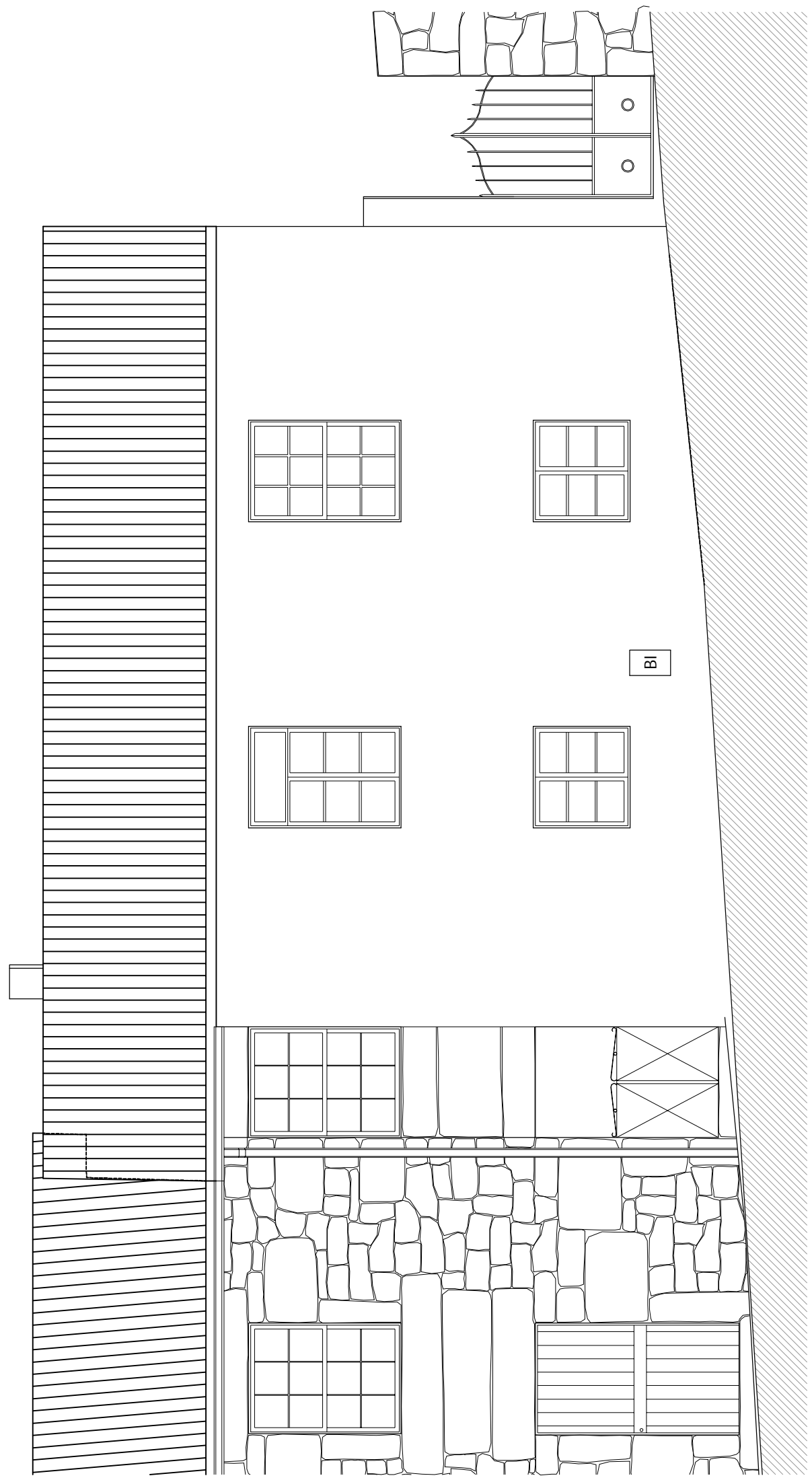
Alçado Nascente
